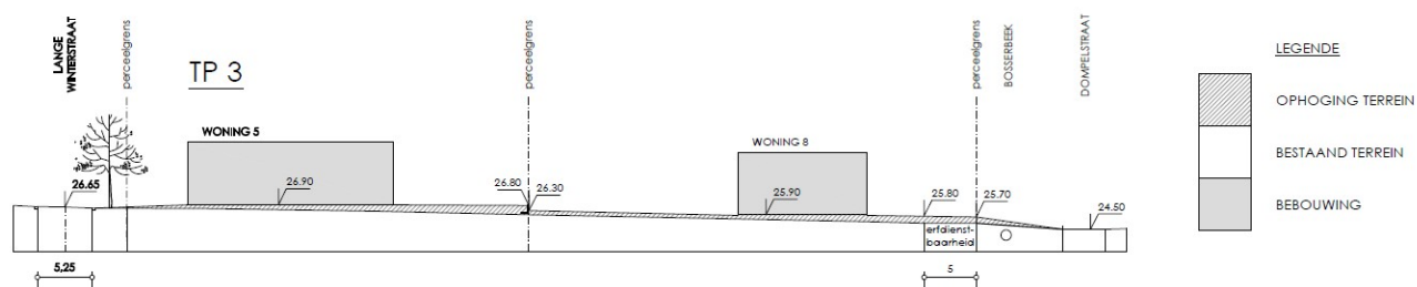
figuur 2. Terreinprofiel van planvoornemen. Bron: Architectenbureau JO JANSSENS, dossier 201607, d.d. 20-9-2016.
