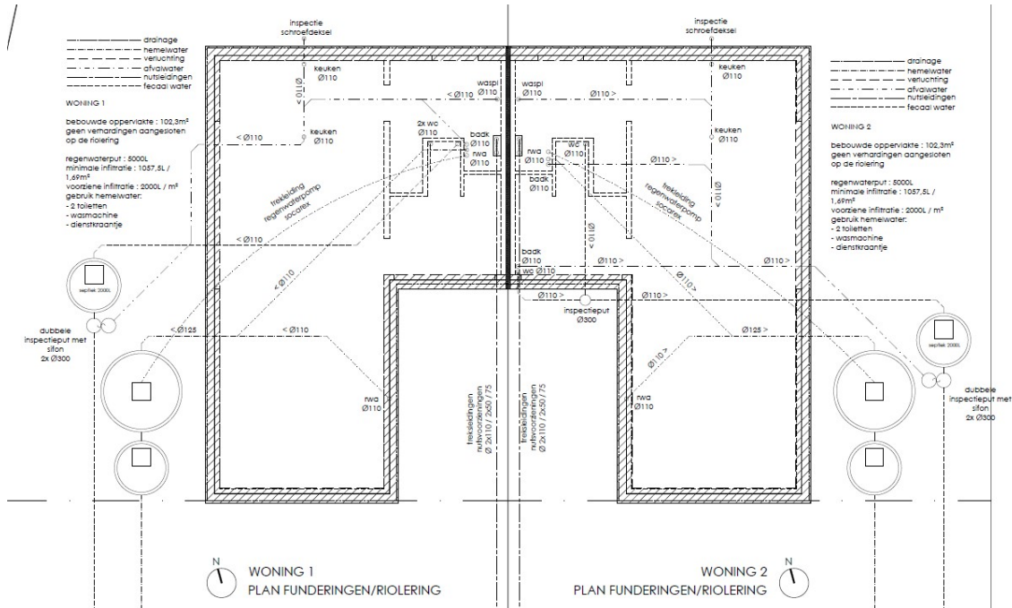
figuur 4. Plattegrond (funderings- en rioleringsplan) van woning 1 en 2. Bron: Architectenbureau JO JANSSENS, dossier 201607, d.d. 20-9-2016.
