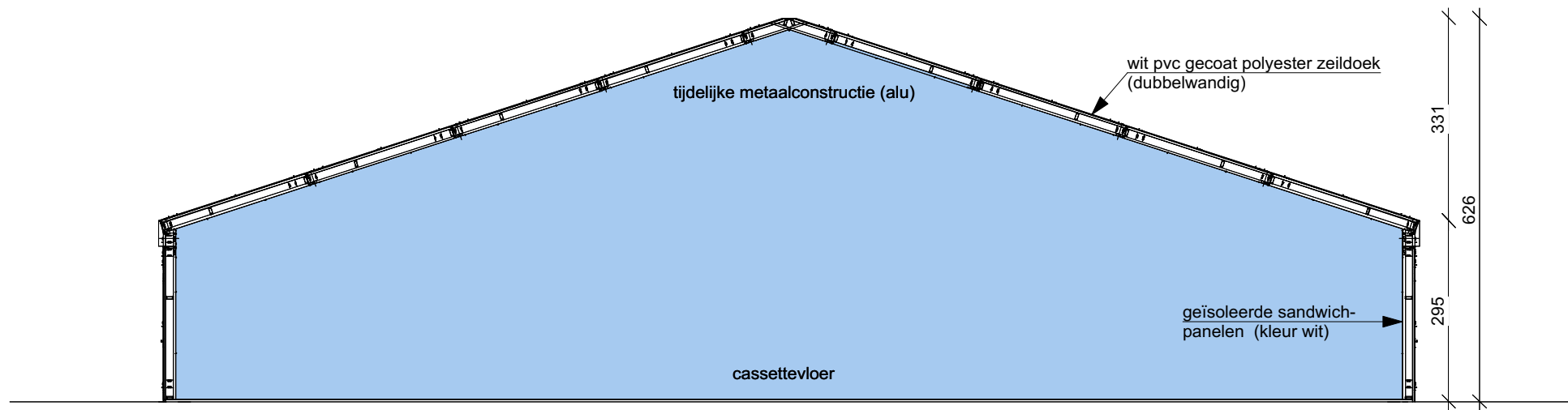
VERTIKALE SNEDE aa schaal 1/100
