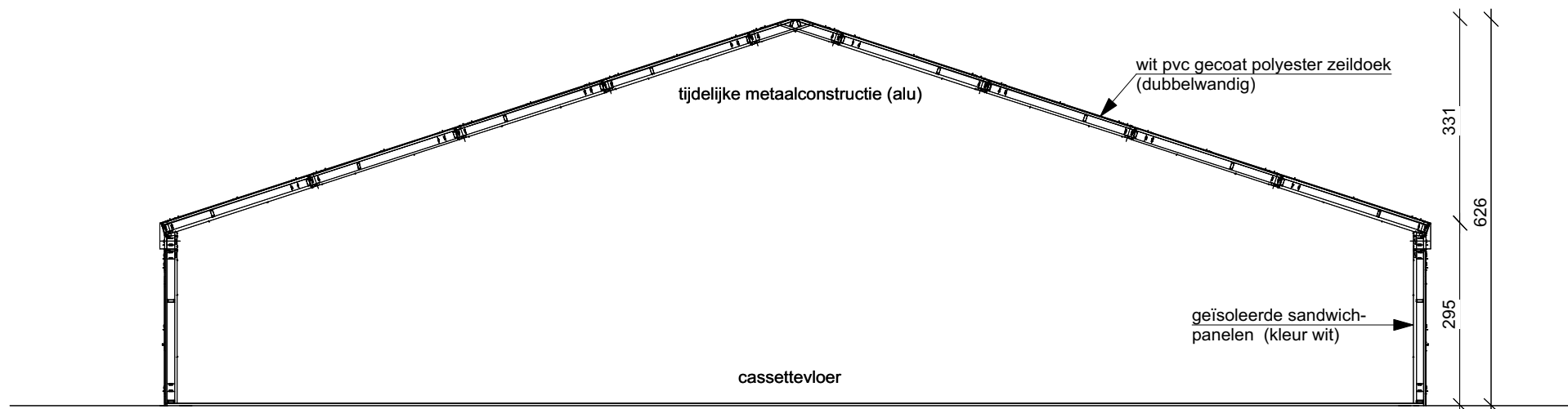
VERTIKALE SNEDE aa schaal 1/100
