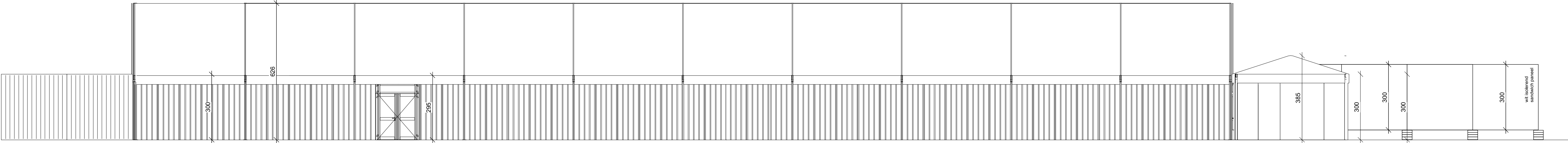
ZUIDgevel schaal 1/100
