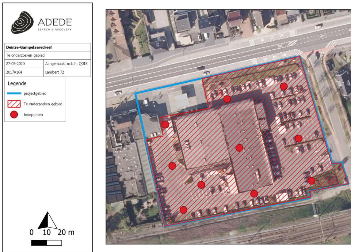
Figuur 2. Boorplan
