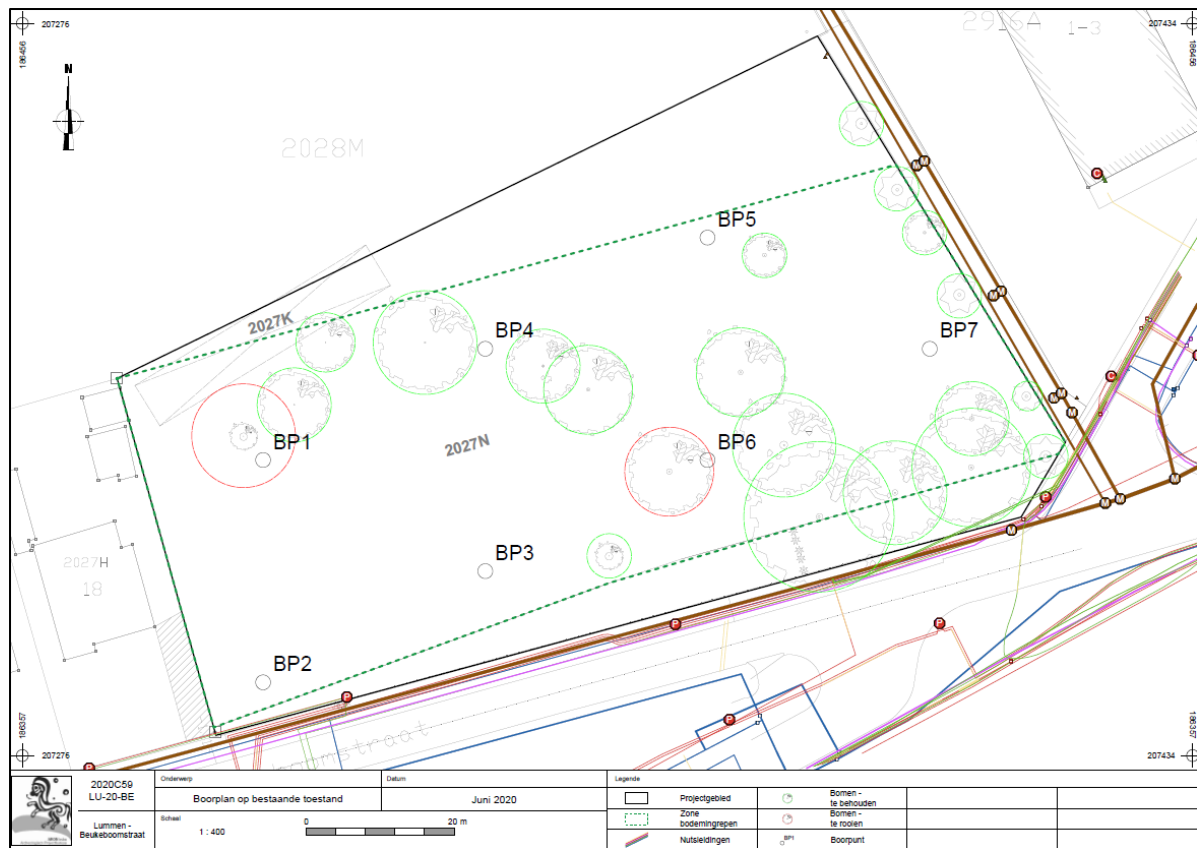
Afb. 28: Boorplan met aanduiding van de boorpunten, het projectgebied (zwart) en de zone voor vervolgonderzoek (groen) op bestaande toestand (BT), met te behouden (groen) en te rooien bomen (rood) (Bron: Aron bv, digitaal plan, dd. 16/06/2020, aanmaatschaal 1.400, 2020C59).
