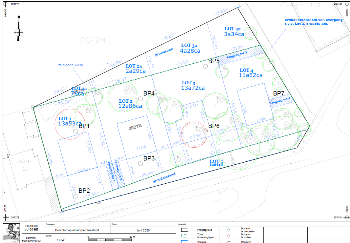
Afb. 29: Boorplan met aanduiding van de boorpunten, het projectgebied (zwart) en de zone voor vervolgonderzoek (groen) op ontworpen toestand (OT), met te behouden (groen) en te rooien bomen (rood) (Bron: Aron bv, digitaal plan, dd. 16/06/2020, aanmaatschaal 1.400, 2020C59).
