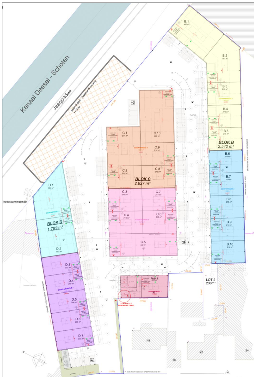
Afb. 3. Inplantingsplan van de nieuwe leidingen en infiltratiebekkens onder de verharding.
