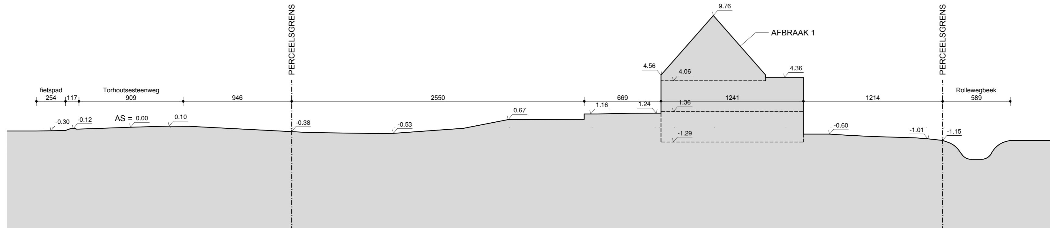
TERREINPROFIEL 1 - bestaande toestand (hoogtepeilen t.o.v. as Torhoutsesteenweg)
