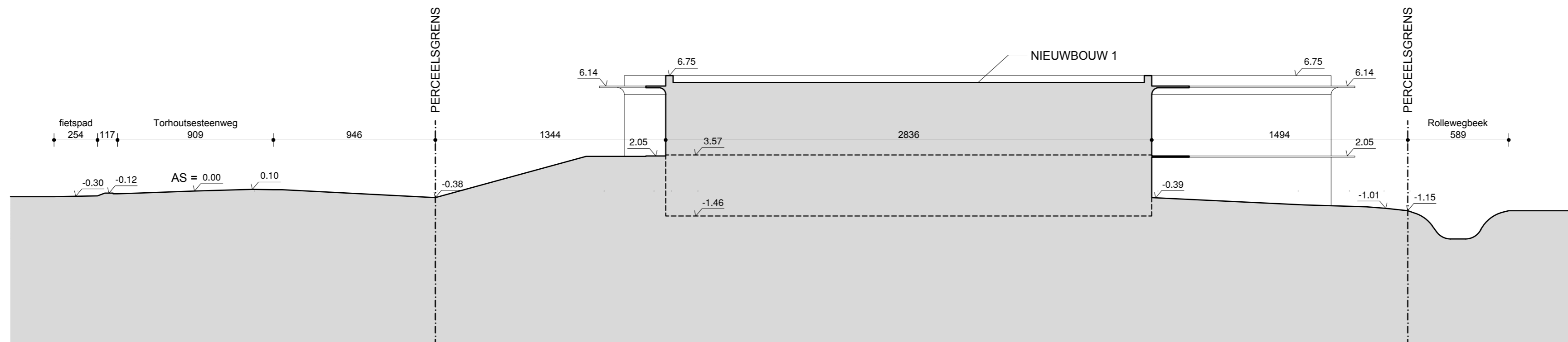
TERREINPROFIEL 1 - nieuwe toestand (hoogtepeilen t.o.v. as Torhoutsesteenweg)
