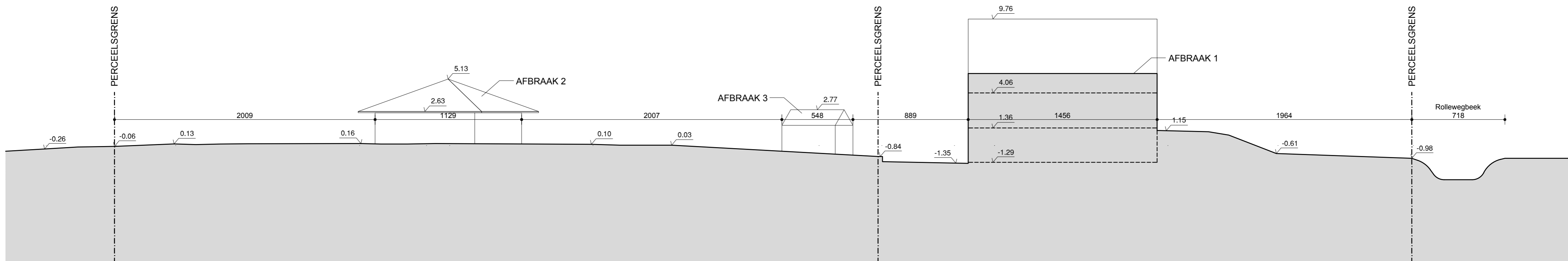
TERREINPROFIEL 2 - bestaande toestand (hoogtepeilen t.o.v. as Torhoutsesteenweg)
