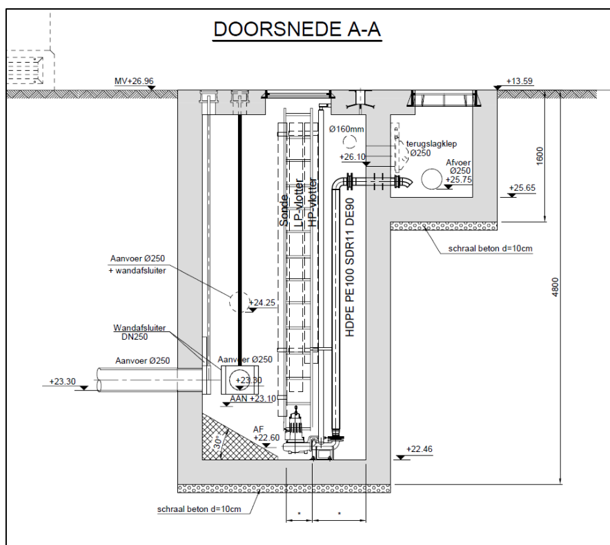
Figuur 6: Doorsnede PS 1. (Bron: initiatiefnemer, 2019).
