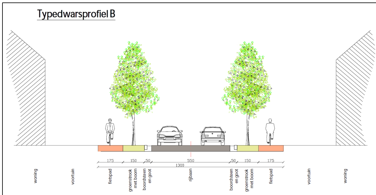
Figuur 8: Typedwarsprofiel St.-Apolloniaalaan. (Bron: initiatiefnemer, 2019).
