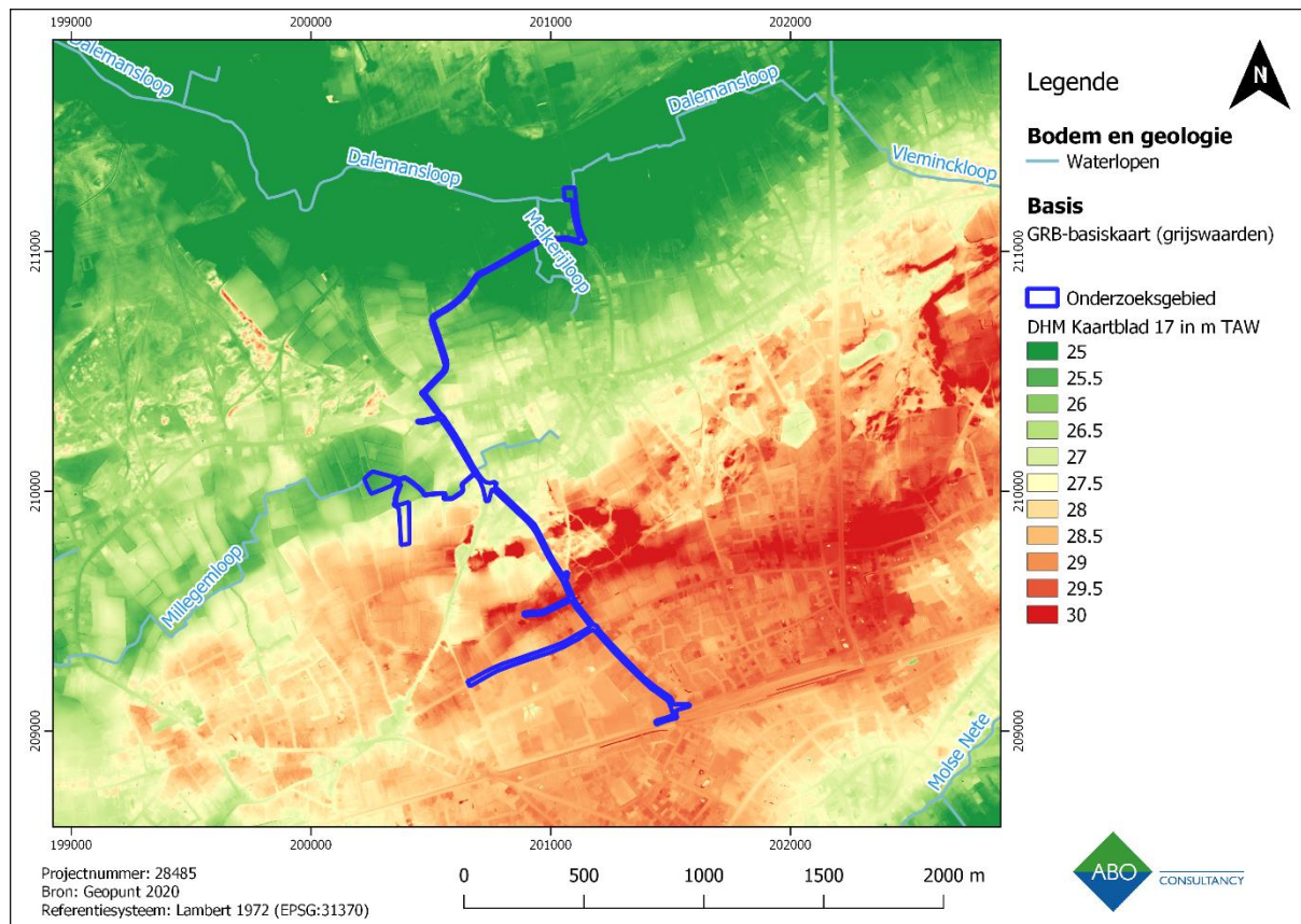
Figuur 13: Digitaal Hoogtemodel (DHMVII) (1m) met aanduiding van het projectgebied in detail. (Bron: Geopunt, 2019)
