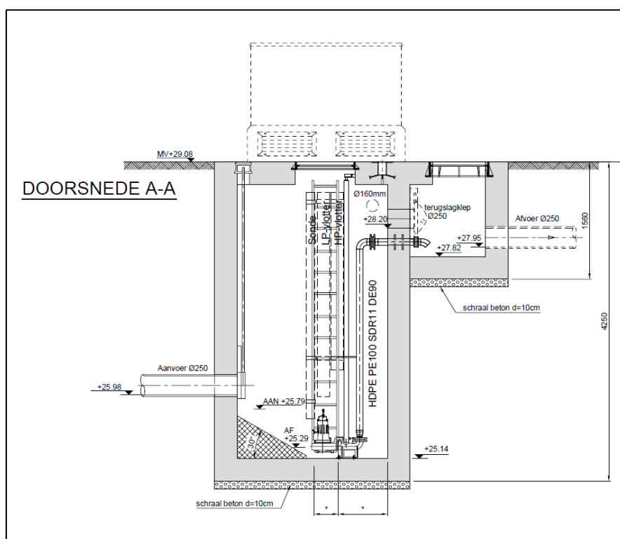
Figuur 7: Doorsnede PS 2. (Bron: initiatiefnemer, 2019).
