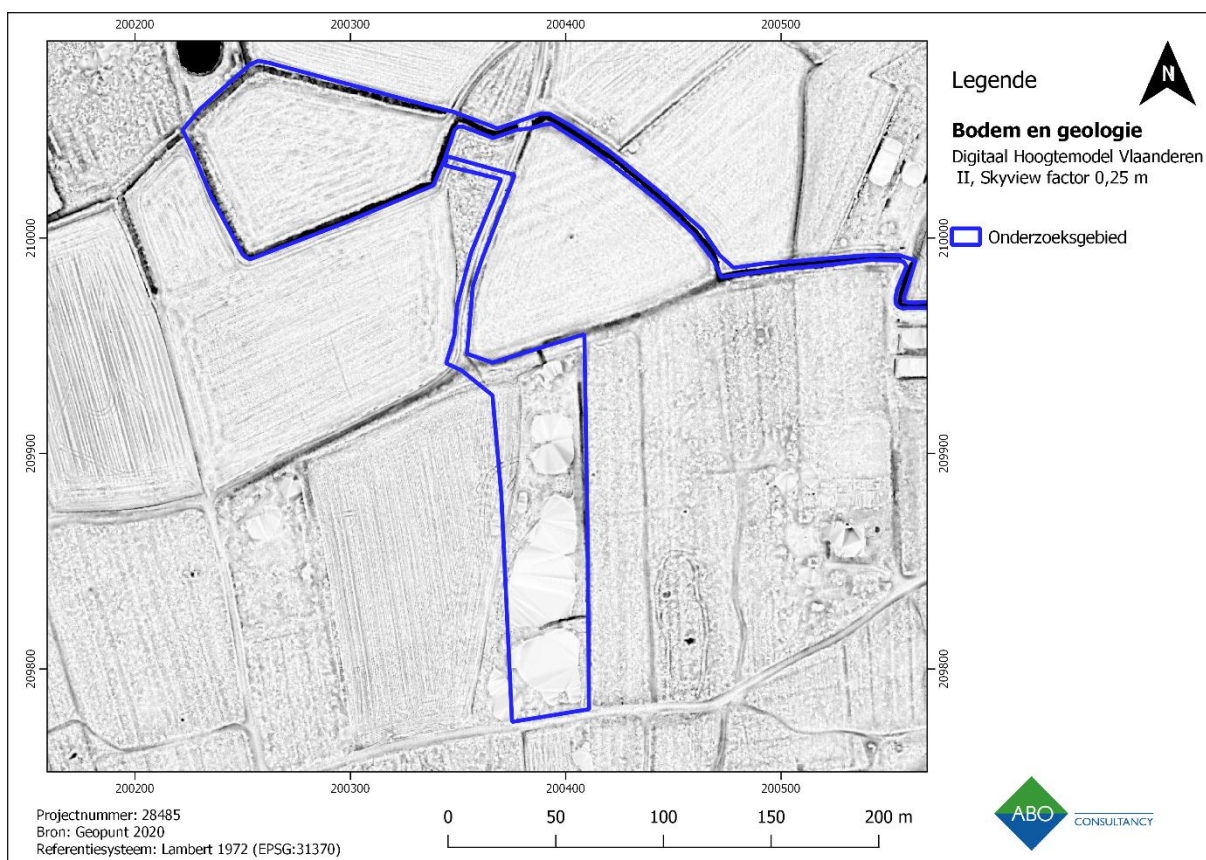
Figuur 18: Skyview (0,25m) met aanduiding van het projectgebied, detail Demerloop. (Bron: Geopunt, 2019)
