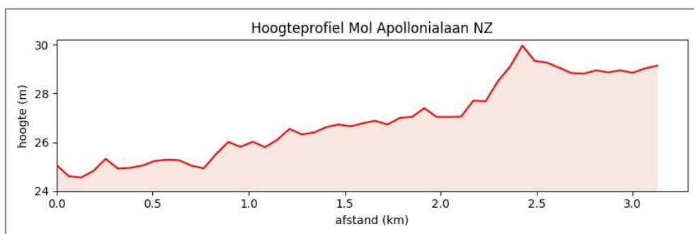
Figuur 14: Hoogteprofiel ZN. (Bron: Geopunt, 2019)
