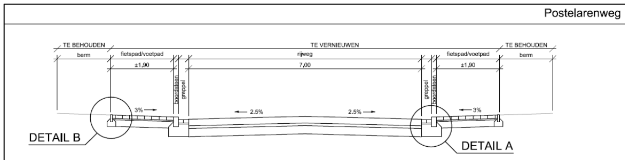
Figuur 9: Typedwarsprofiel St.-Apolloniaalaan. (Bron: initiatiefnemer, 2019).
