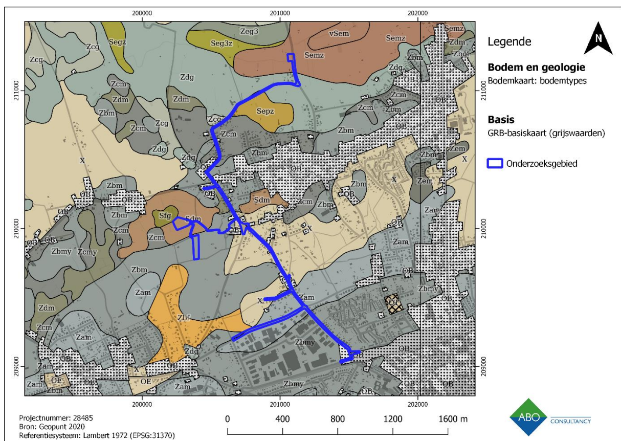
Figuur 19: Gedigitaliseerde bodemkaart met aanduiding van het projectgebied. (Bron: Geopunt, 2019)
