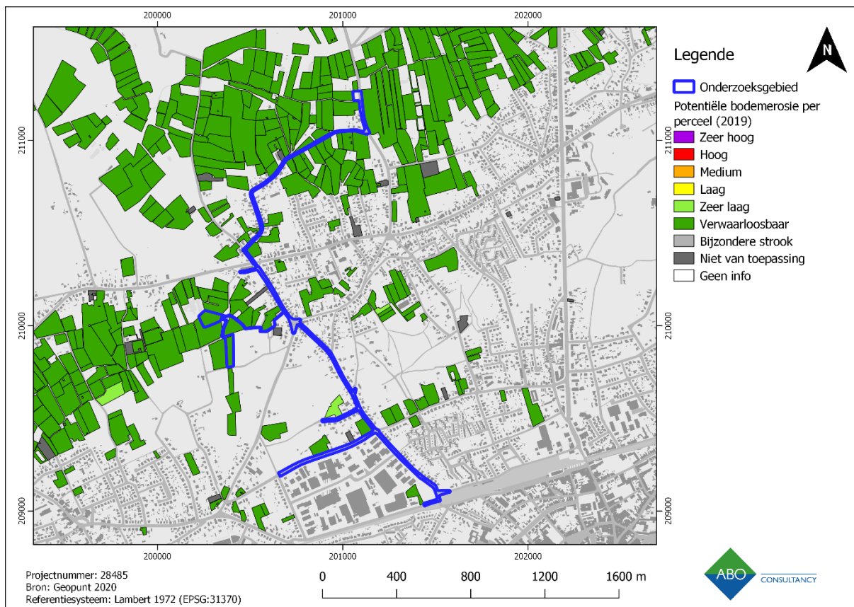
Figuur 24: Bodemerosiekaart op perceelniveau met aanduiding van het projectgebied. (Bron: Geopunt, 2019)
