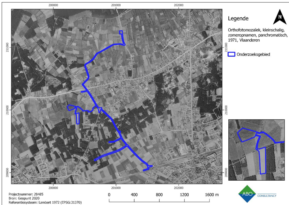
Figuur 34: Orthofotomozaïek 1971 met aanduiding van het projectgebied. (Bron: Geopunt, 2019)
