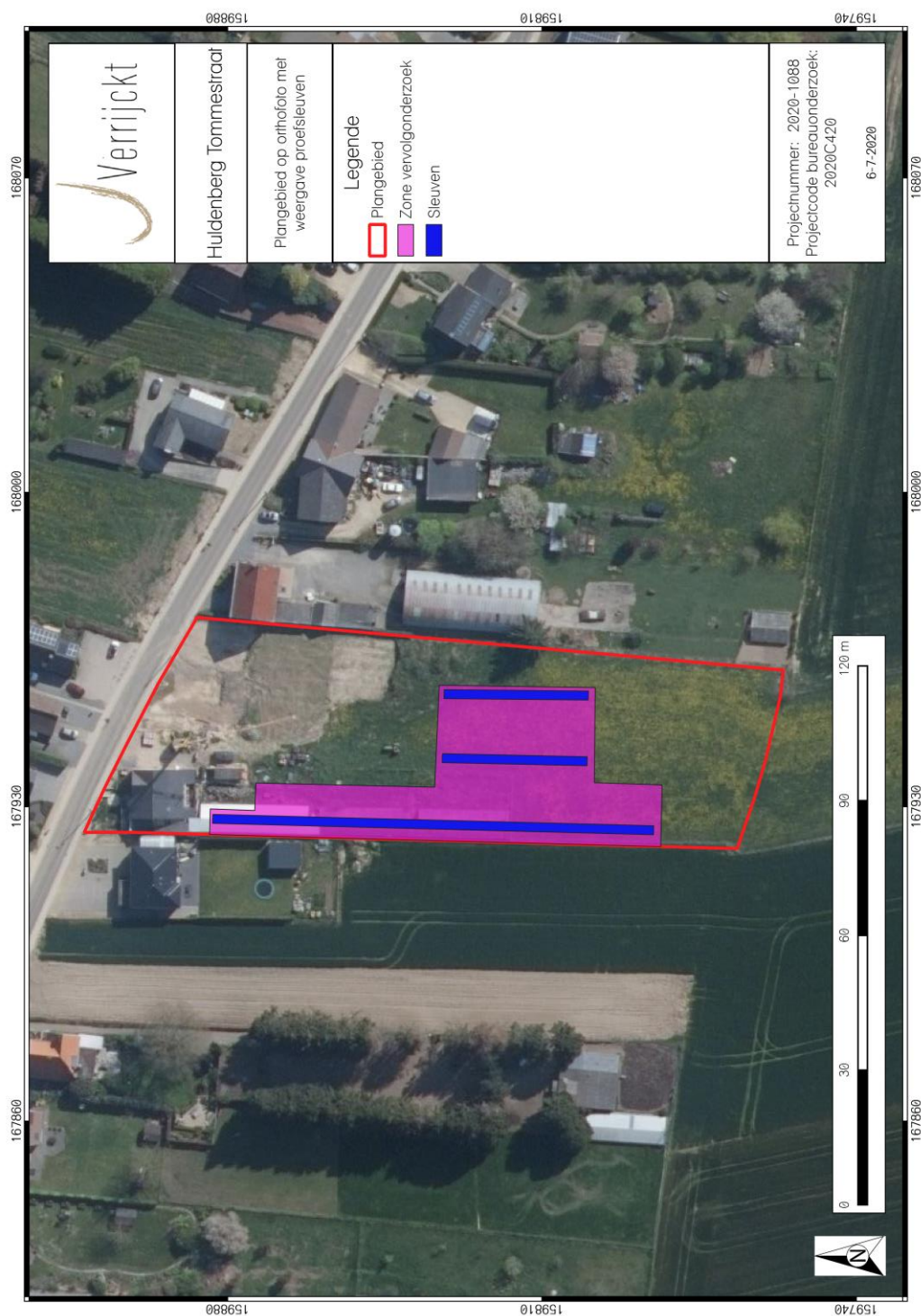
Figuur 3: Sleuvenplan
