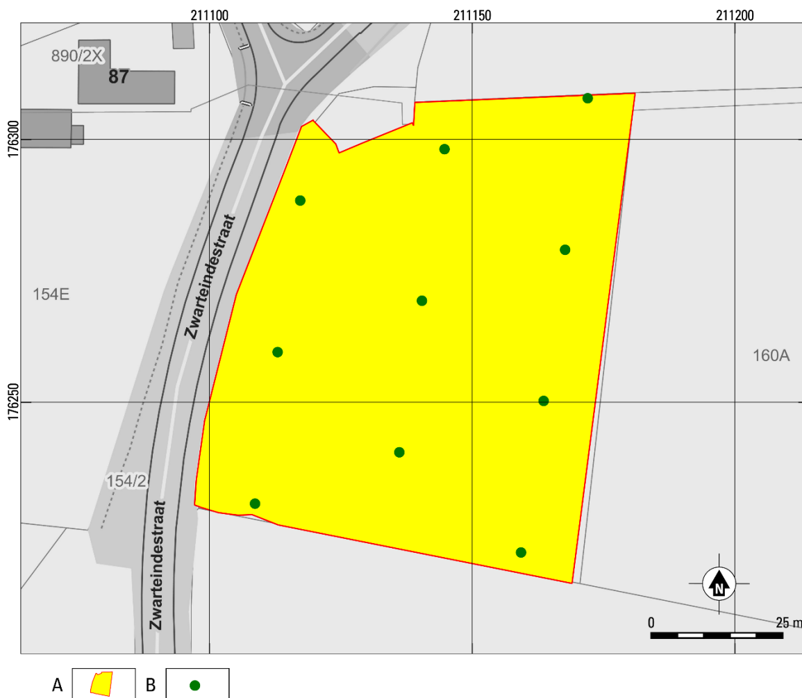
Fig. 3. Nieuwerkerken – Riolerings- en wegniswerken Zwarteindestraat-Doorstraat (21.896V). Indicatie van de geplande landschappelijke boringen.
