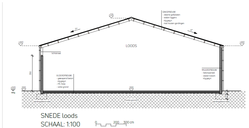
Figuur 4: Snede loods (LV-architecten bvba en DLV Turnhout, 2020)
