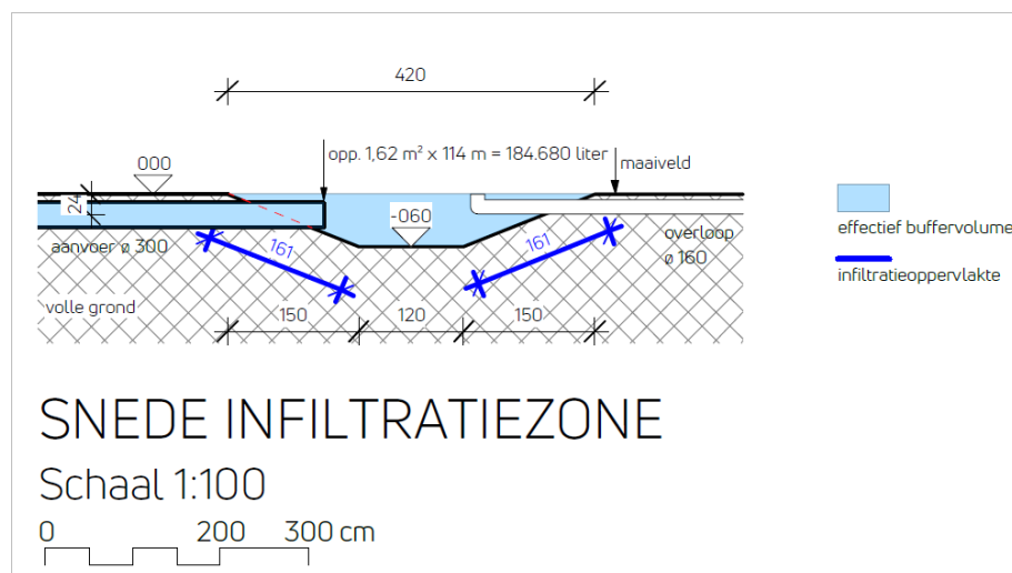
Figuur 5: Snede infiltratiezone (LV-architecten bvba en DLV Turnhout, 2020)
