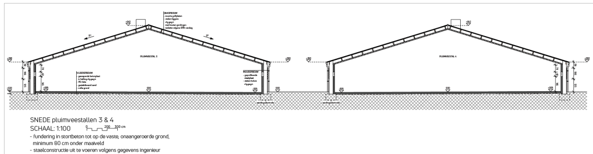
Figuur 3: Snede pluimveestallen (LV-architecten bvba en DLV Turnhout, 2020)
