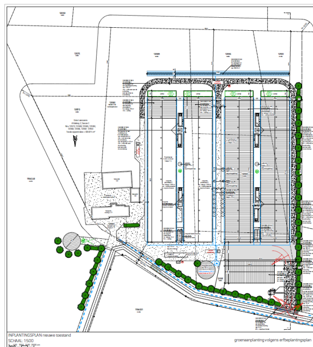
Figuur 2: Inplanting (LV-architecten bvba en DLV Turnhout, 2020)
