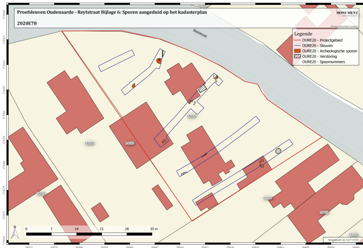
Figuur 1: Sporenplan geprojecteerd op het GRB.
