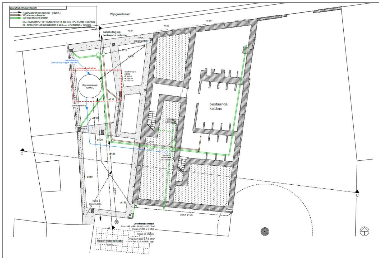
Figuur 7. Funderings- en kelderplan nieuwe toestand.
