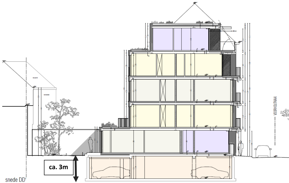
Figuur 9 Doorsnede geplande werken. (bron: opdrachtgever)
