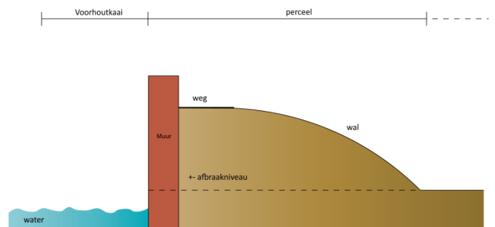
Figuur 41: Schematische voorstelling van de doorsnede van de courtine en de positionering van de huidige kaai en het perceel. Deze vereenvoudigde afbeelding geeft de trefkans weer op resten van de courtine met muur en wal, die zich onder het afbraakniveau bevinden.
