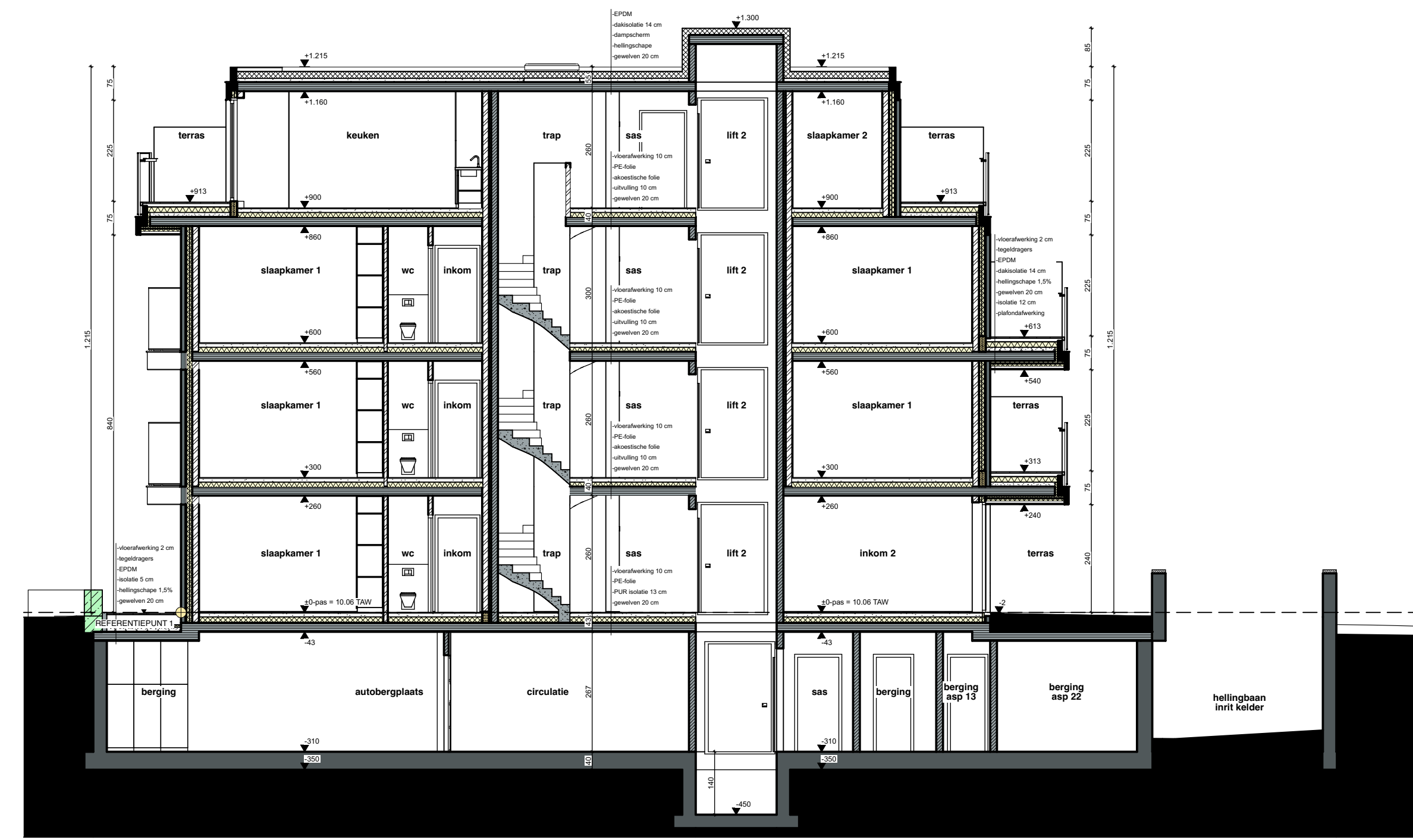
DOORSNEDE 2-2 schaal 1:100 NIEUWE TOESTAND
