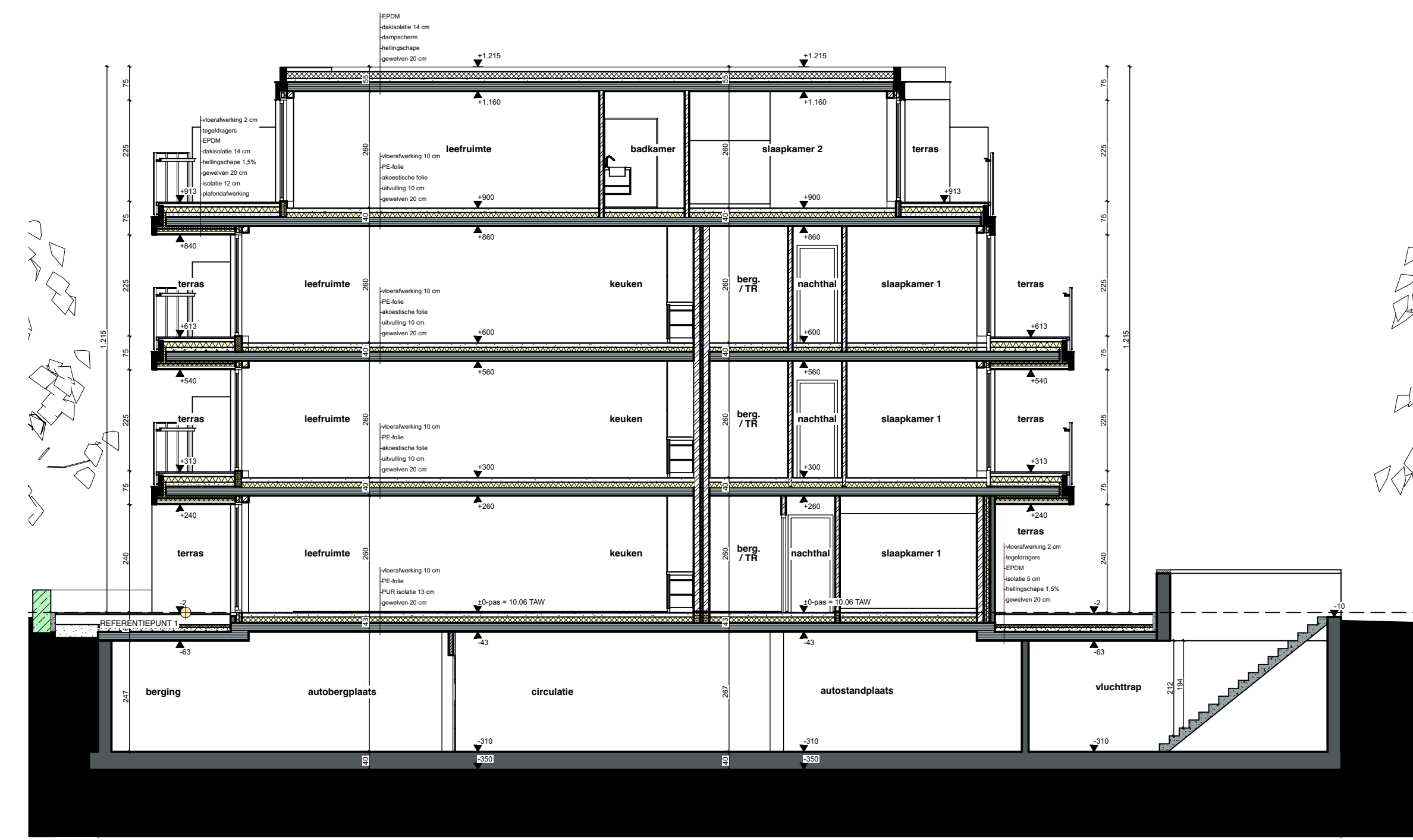
DOORSNEDE 3-3 schaal 1:100 NIEUWE TOESTAND
