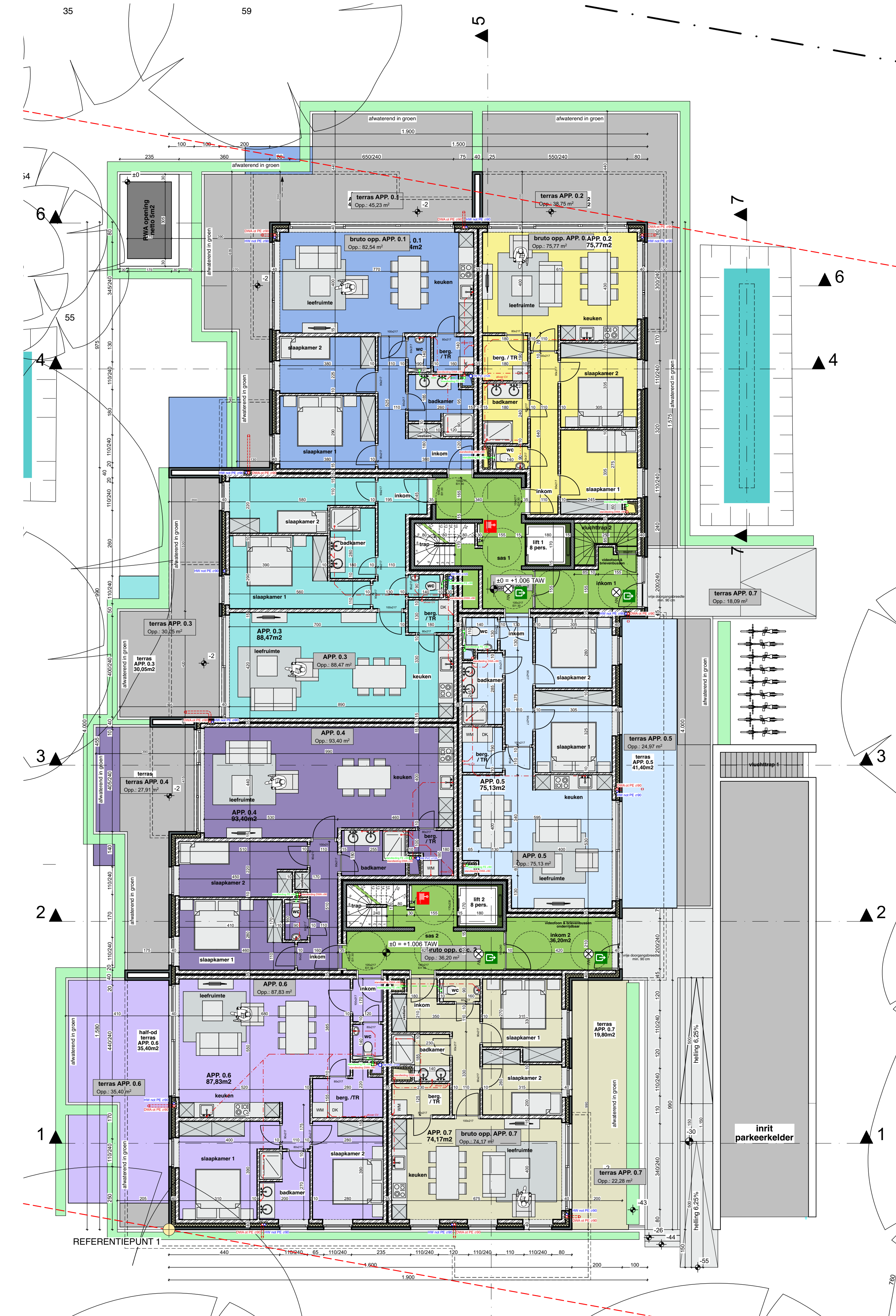
GELIJKVLOERS schaal 1:100 NIEUWE TOESTAND
