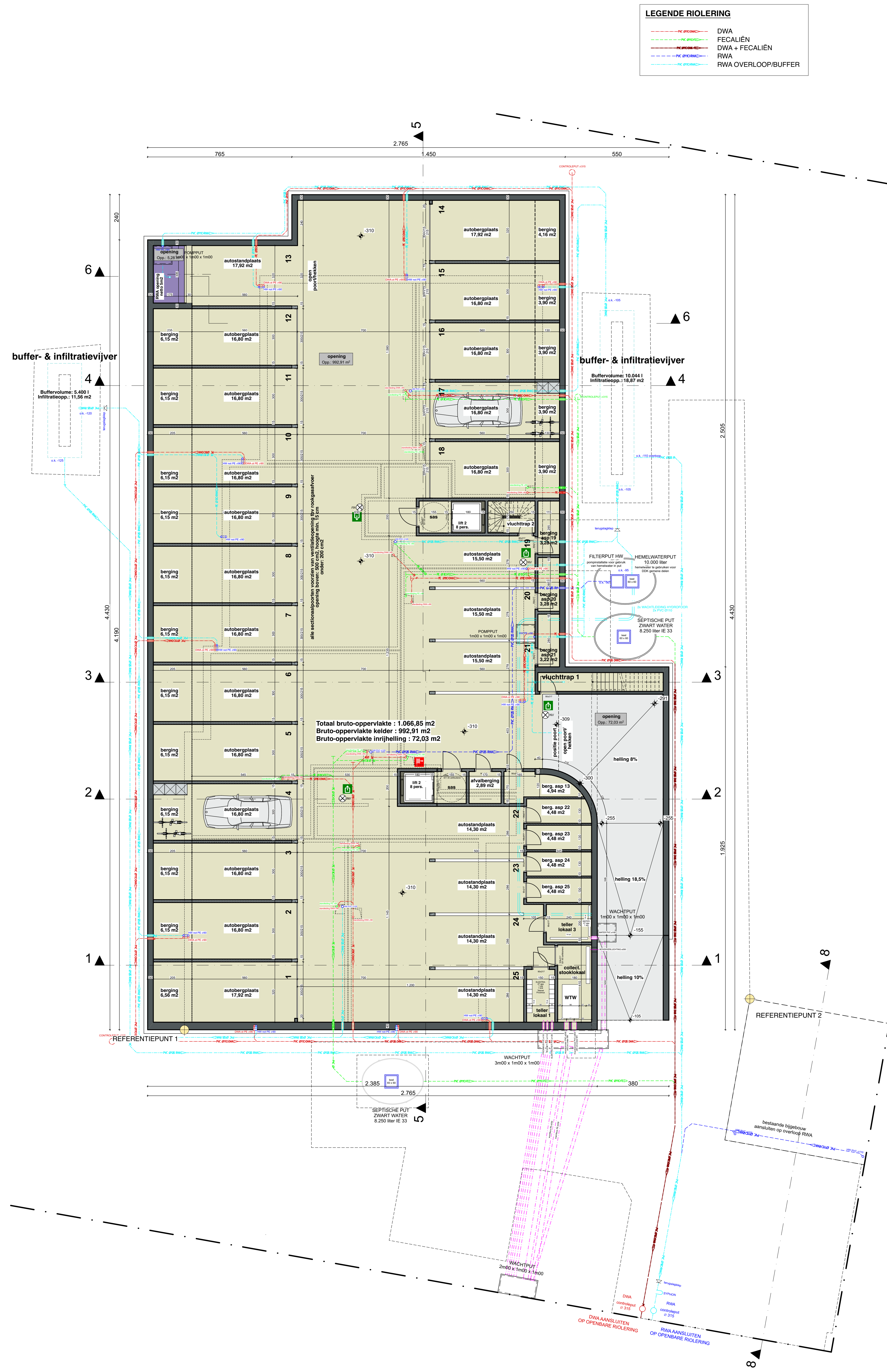
KELDER- & RIOLERINGSPLAN schaal 1:100 NIEUWE TOESTAND
