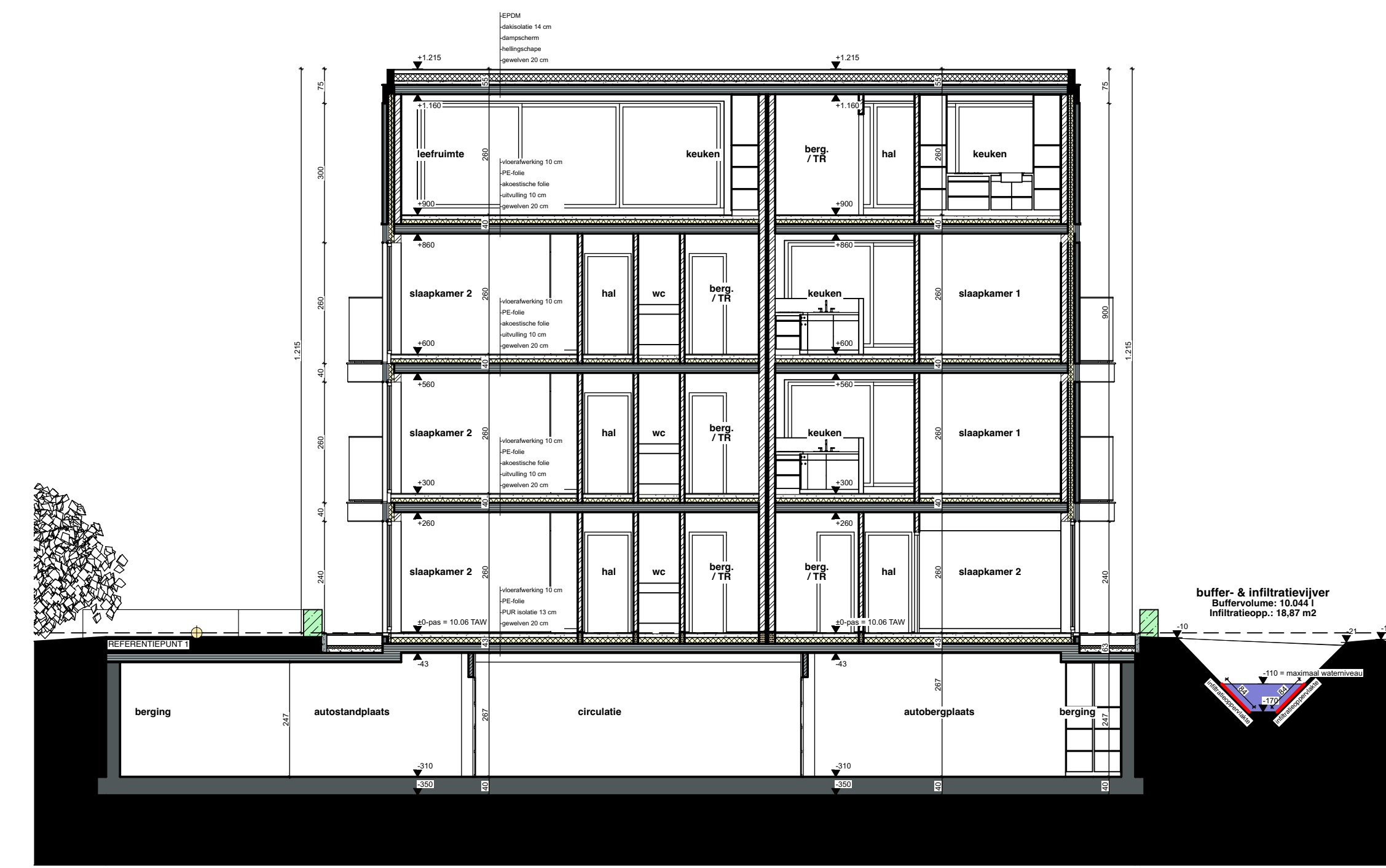
DOORSNEDE 4-4 schaal 1:100 NIEUWE TOESTAND
