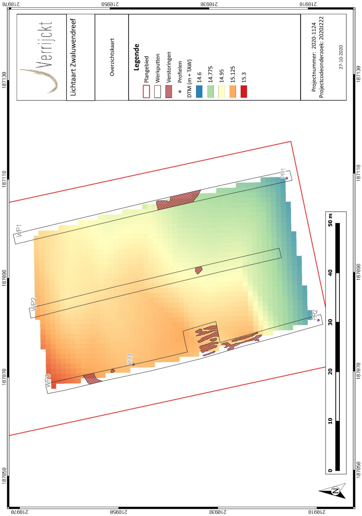
Figuur 1: Syntheseplan
