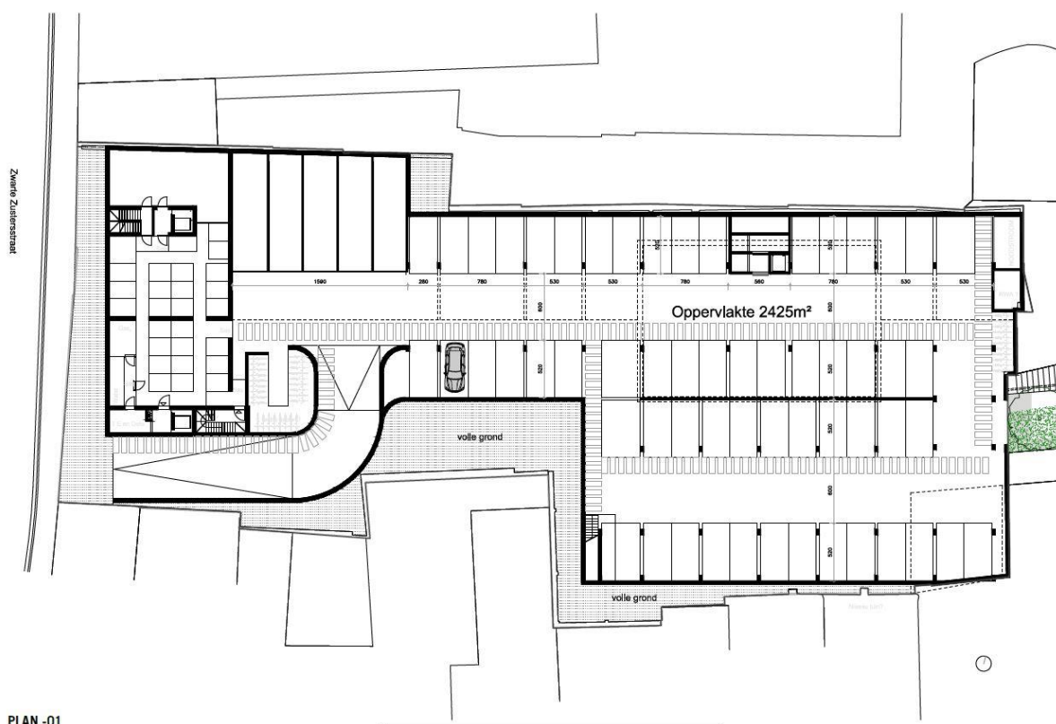
Figuur 42: Nieuw ontwerp ondergronds
