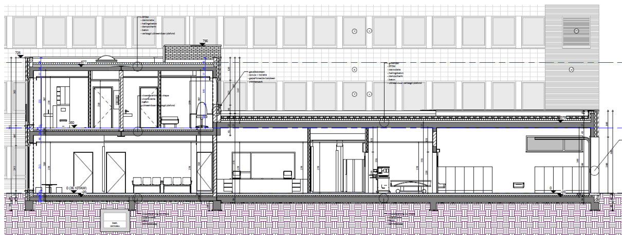
Figuur 14: Sneede B van 'HAP' (Bron: initiatiefnemer, 2019).
