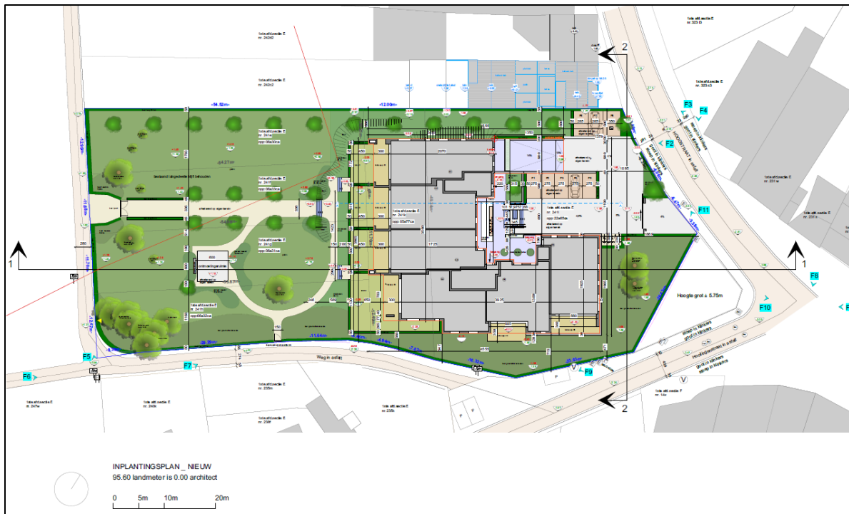
Afb. 3.1: Inplantingsplan met ontworpen toestand (OT) (Bron: Bvba Architectenbureau Houben Philippe, digitaal plan, dd en aanmaatschaal onbekend, 2019E305).
