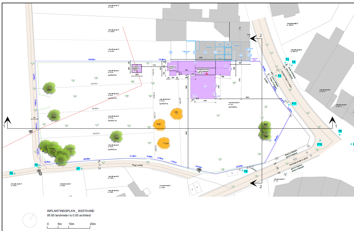
Afb. 3.2: Overzichtsplan met te behouden bomen in het groen en te rooien bomen in het geel. De bebouwing in het paars wordt gesloopt (Bron: Bvba Architectenbureau Houben Philippe, digitaal plan, dd onbekend, aanmaatschaal onbekend, 2019E305)
