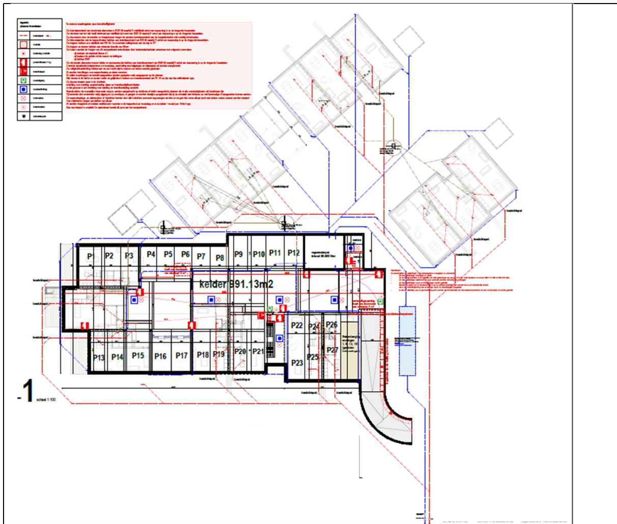
Figuur 4. Grondplan kelder en riolering.
