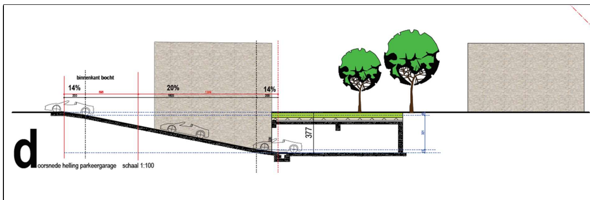
Figuur 5. Doorsnede van de kelder.
