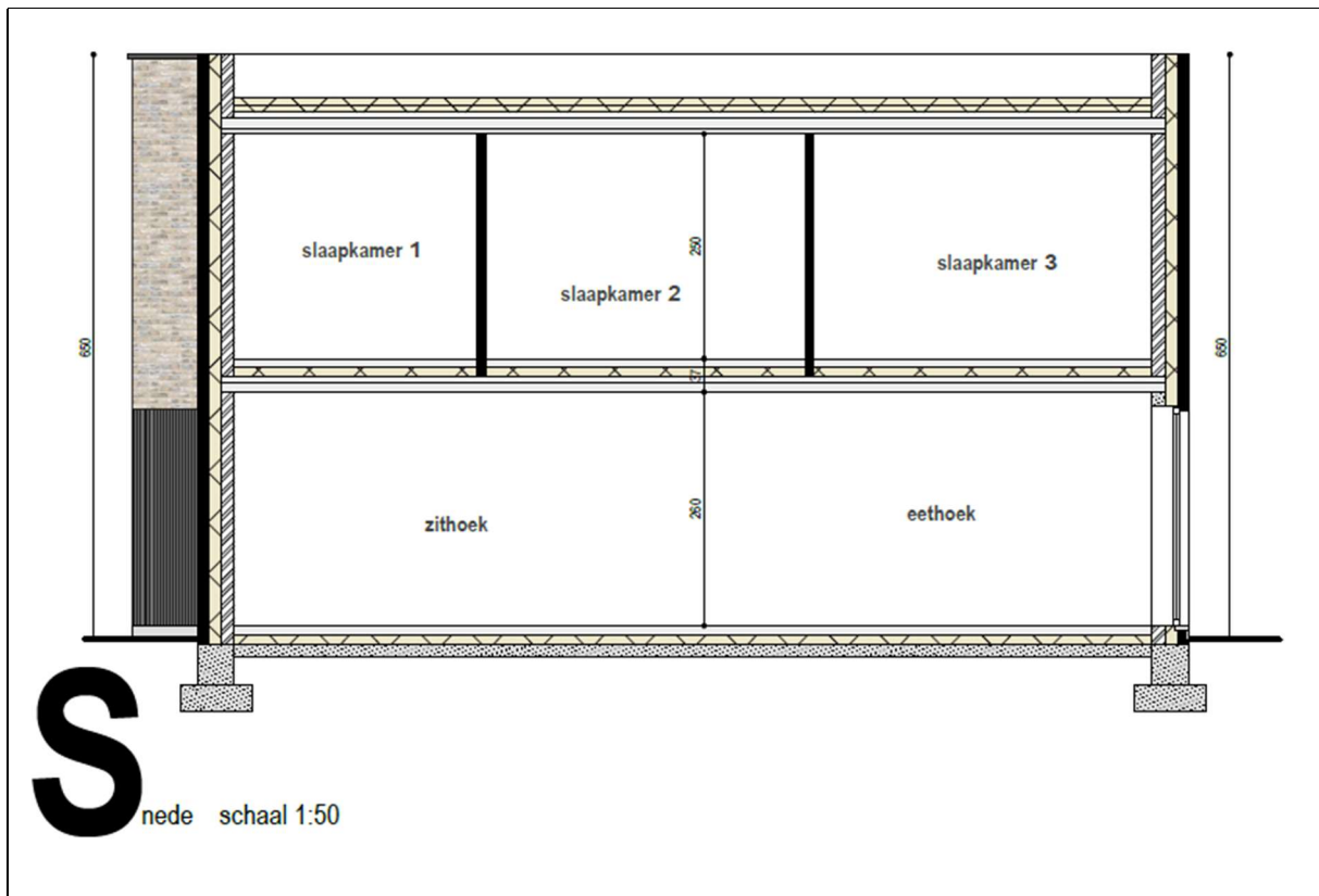
Figuur 6. Typesnede van de ééngezinswoningen.
