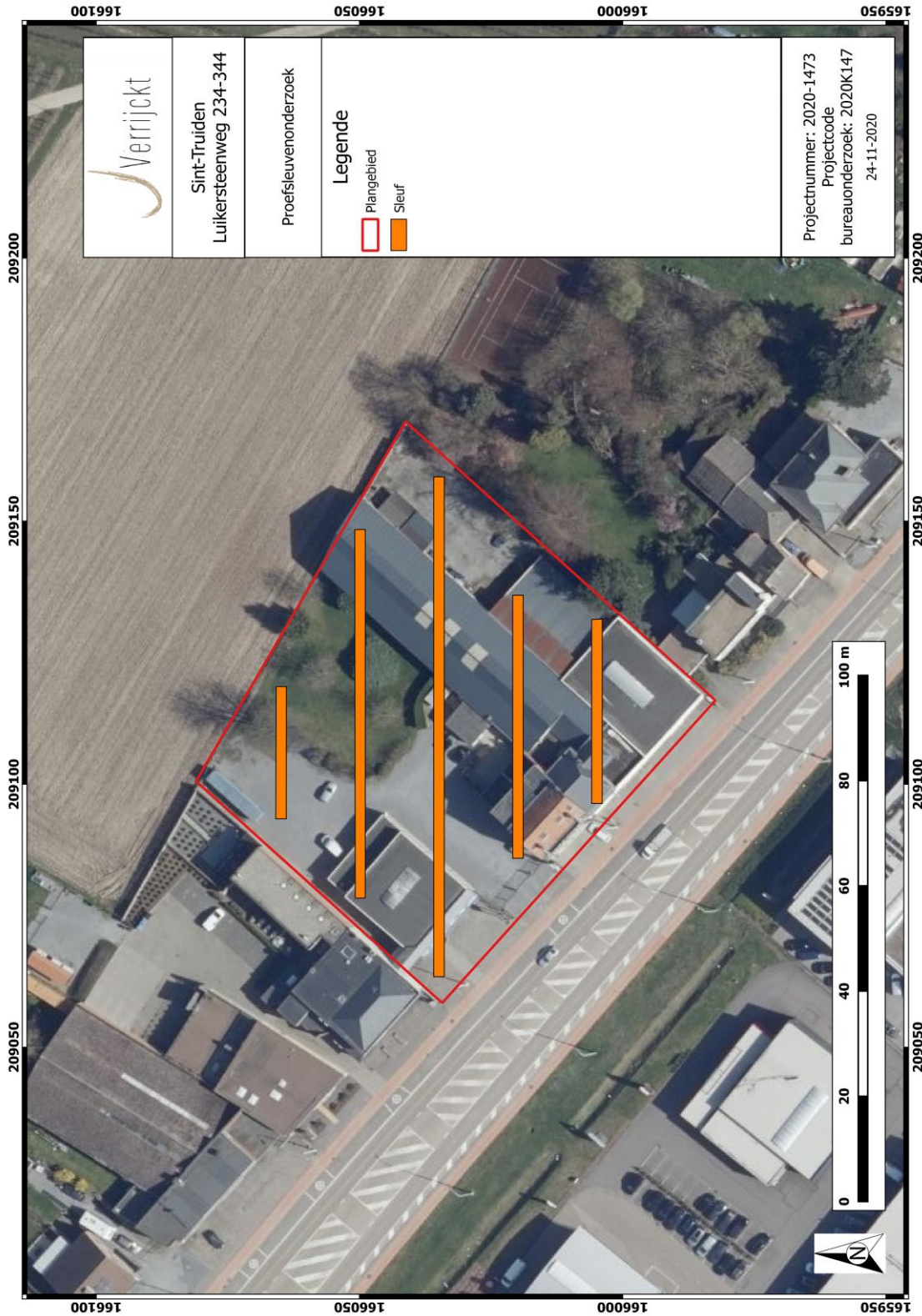
Figuur 4: Sleuvenplan
