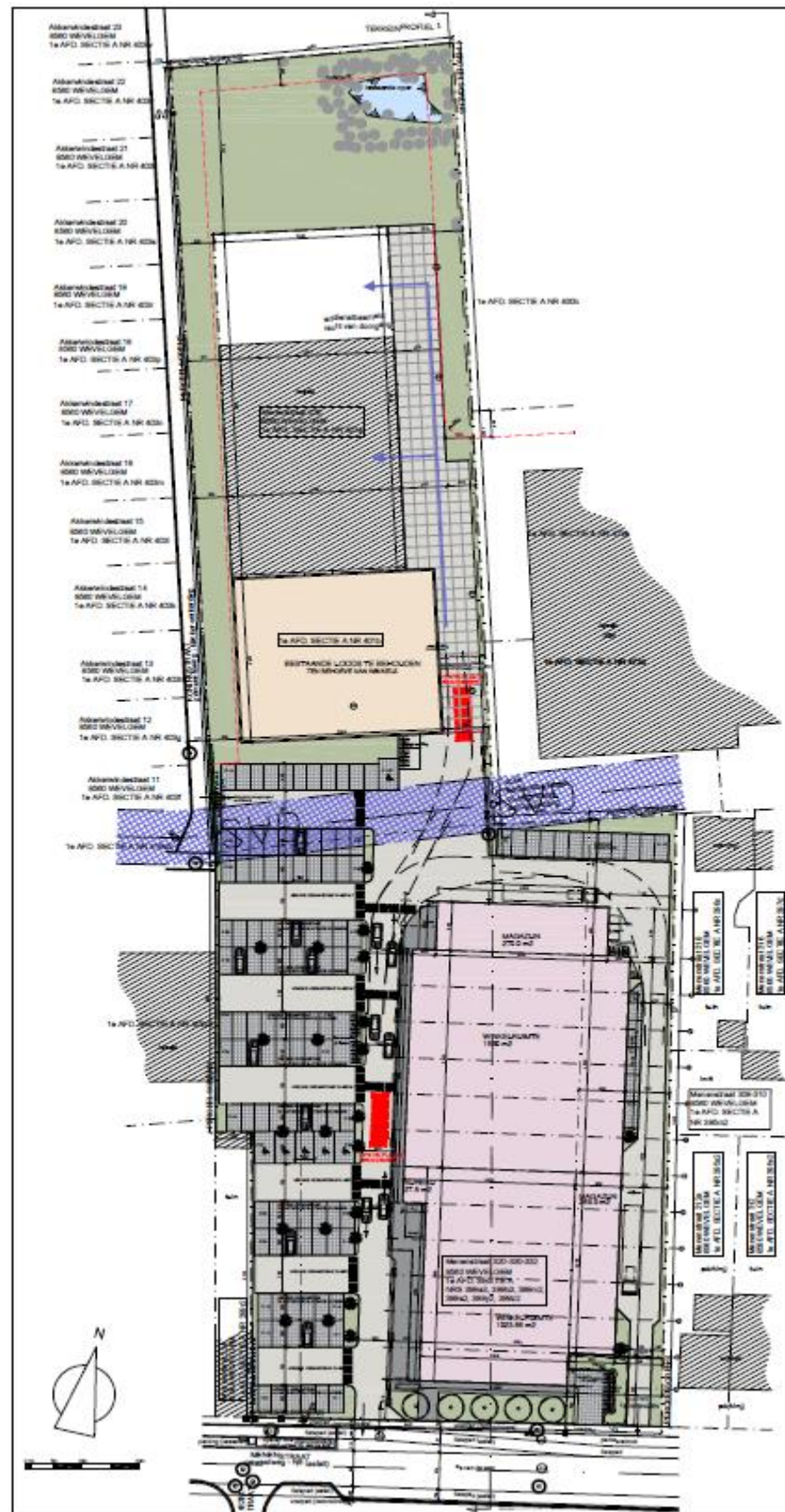
Figuur 13: Inplantingsplan voor de toekomstige situatie (Initiatiefnemer 2020)
