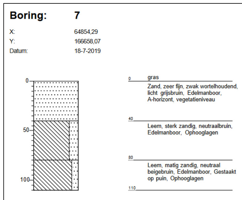
Figuur 53: Boorstaat boring 7 (ABO nv 2019)
