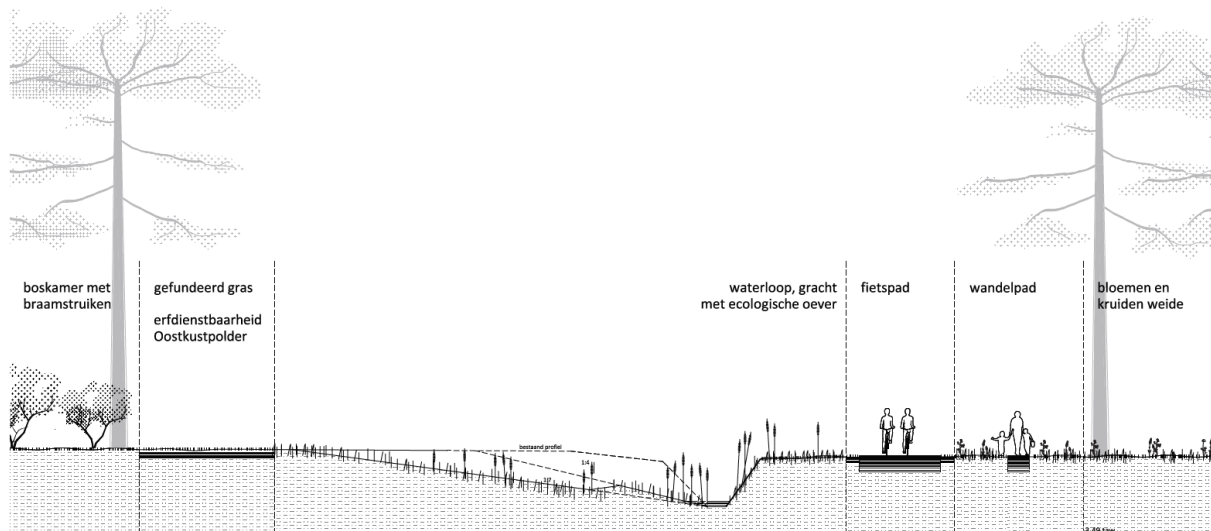
Figuur 3: De geplande dwarsprofielen
