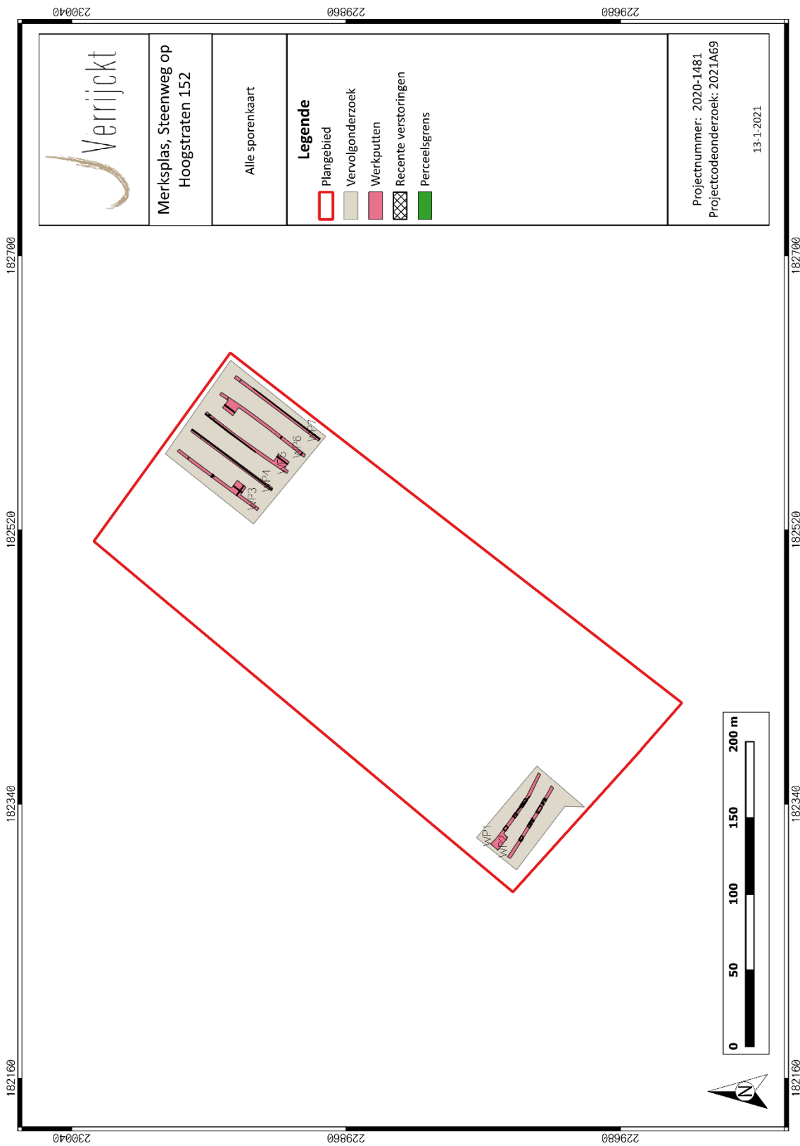
Figuur 1: Syntheseplan
