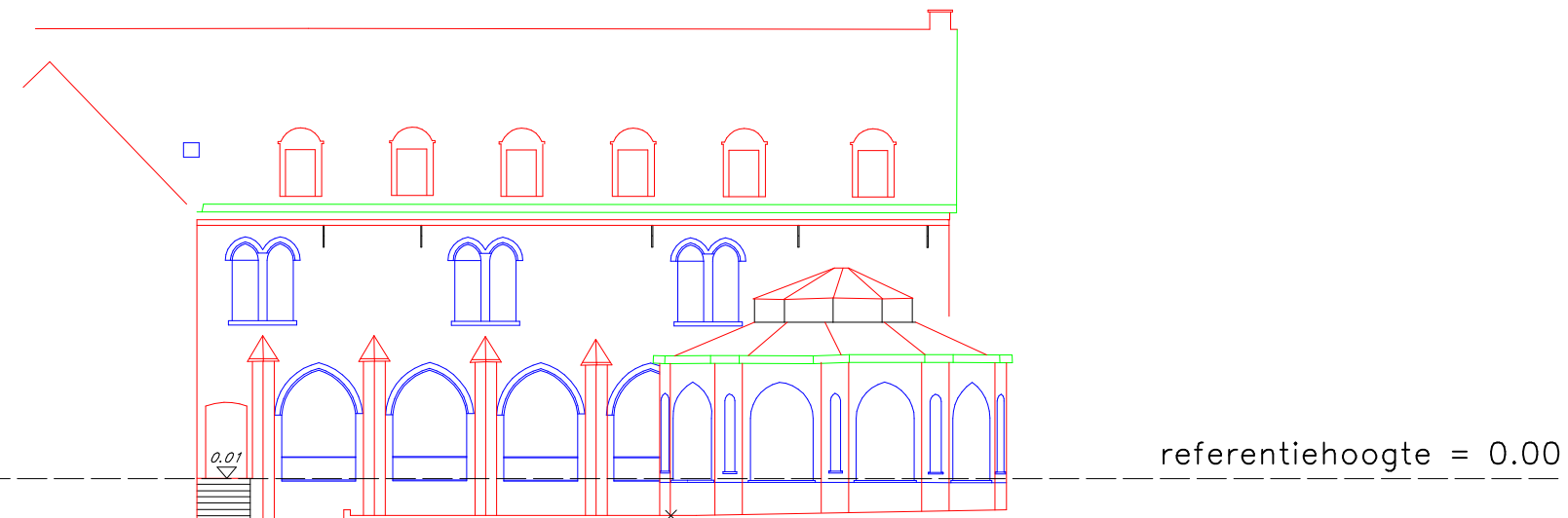
Gevelzicht 4
