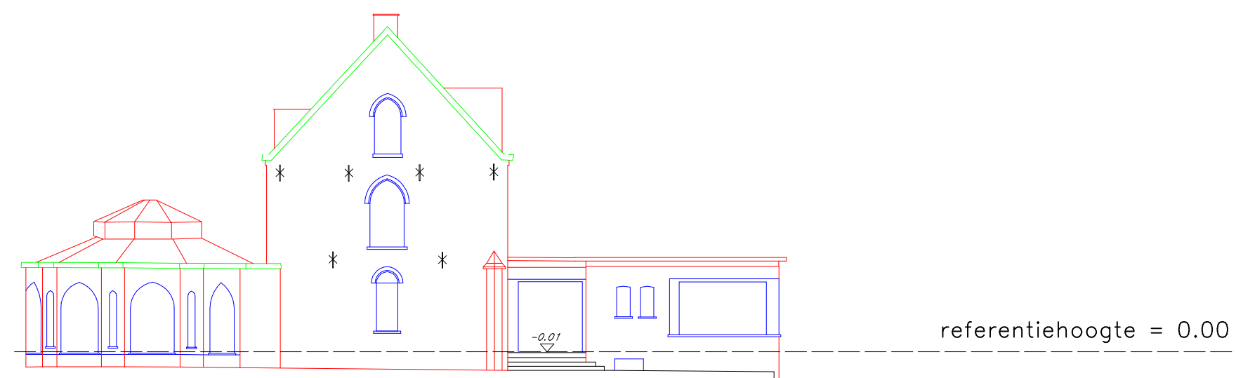
Gevelzicht 6
