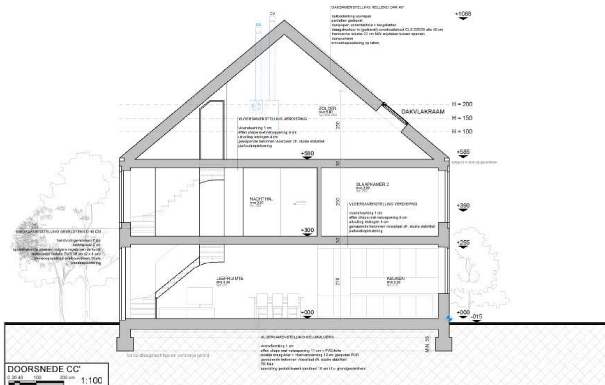
Figuur 10: Typedoorsnede woningen Schrijberg
