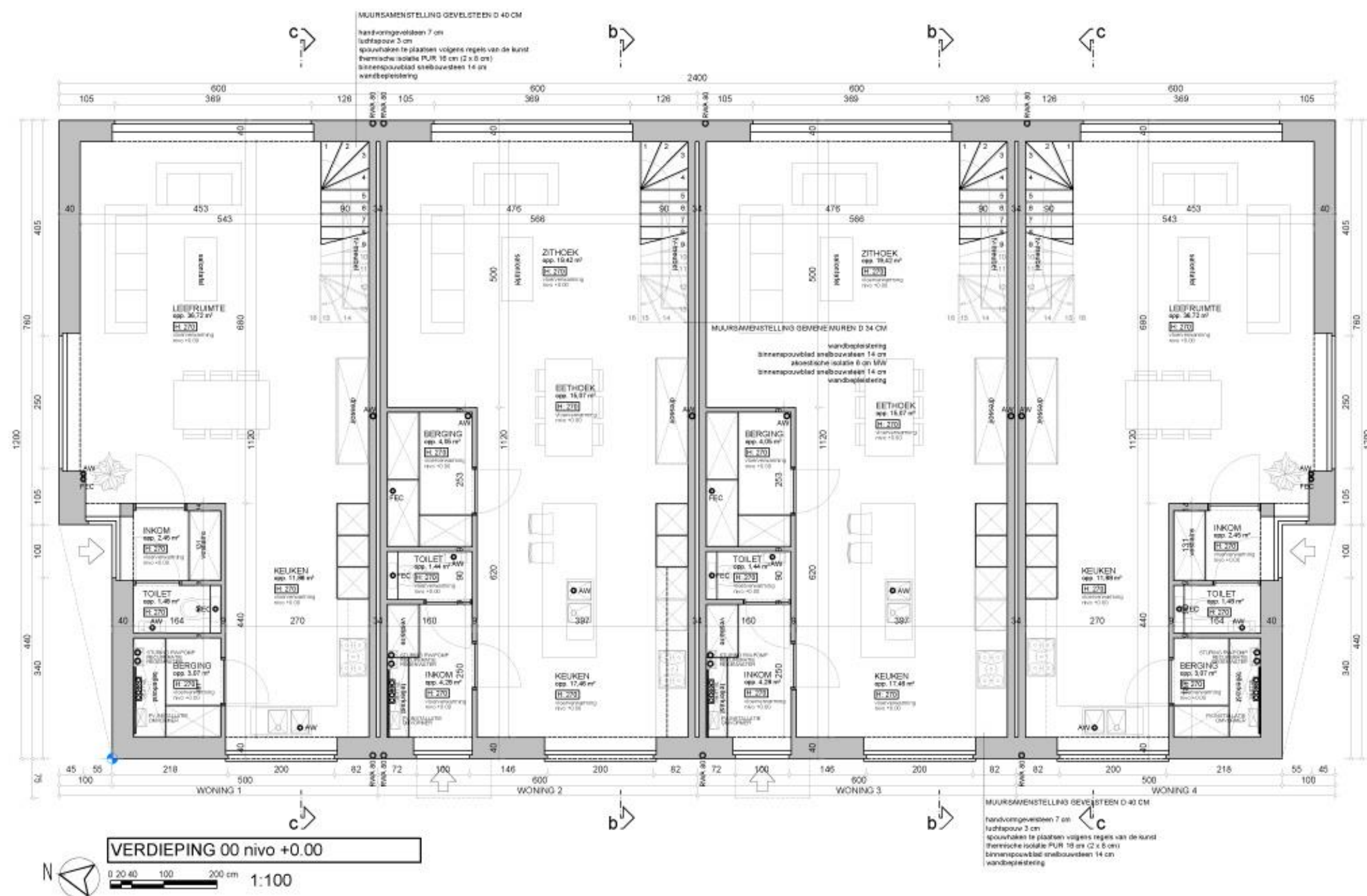
Figuur 8: Grondplan woningen Schrijberg
