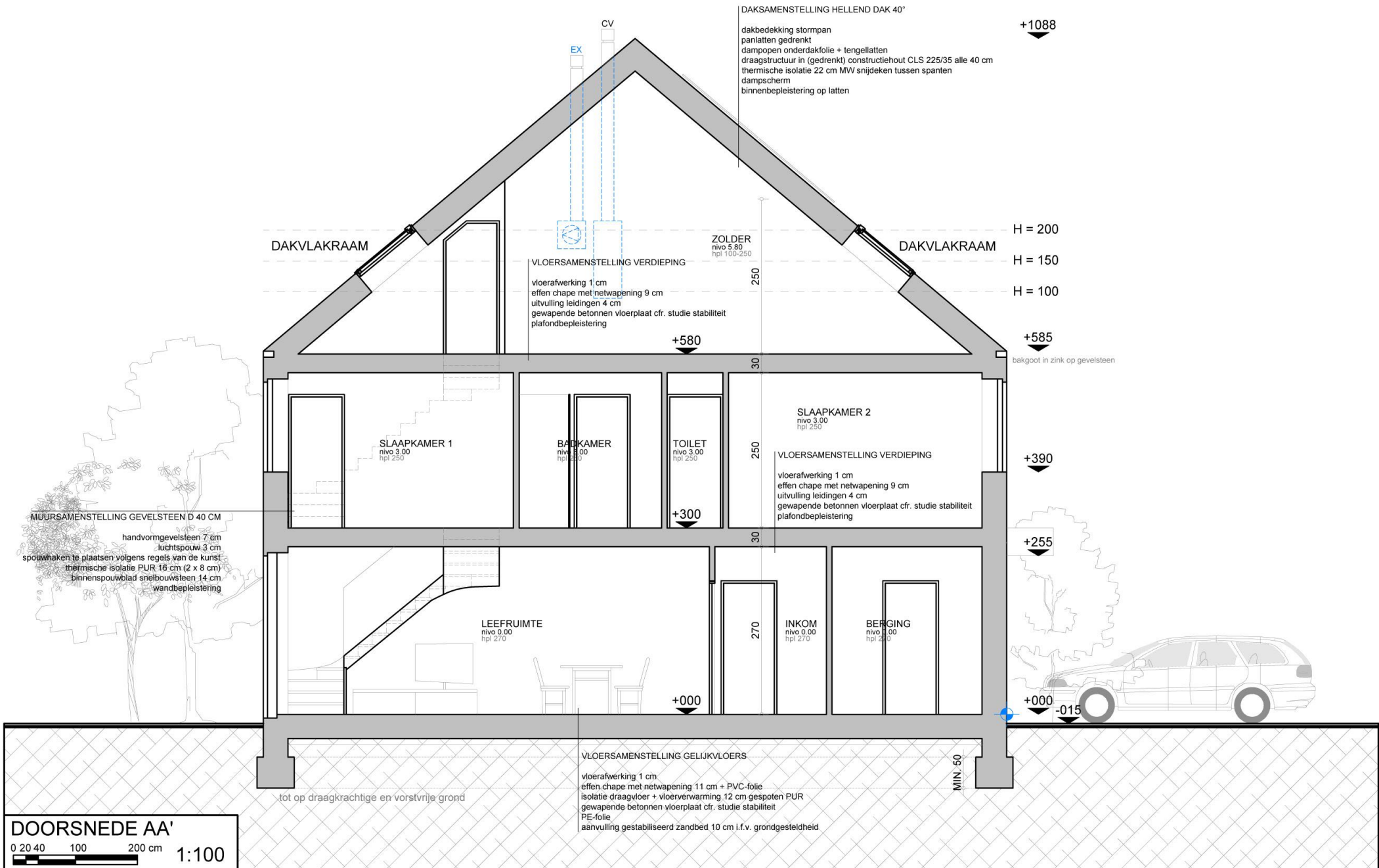
Figuur 7: Typedoorsnede woning Neerkouter
