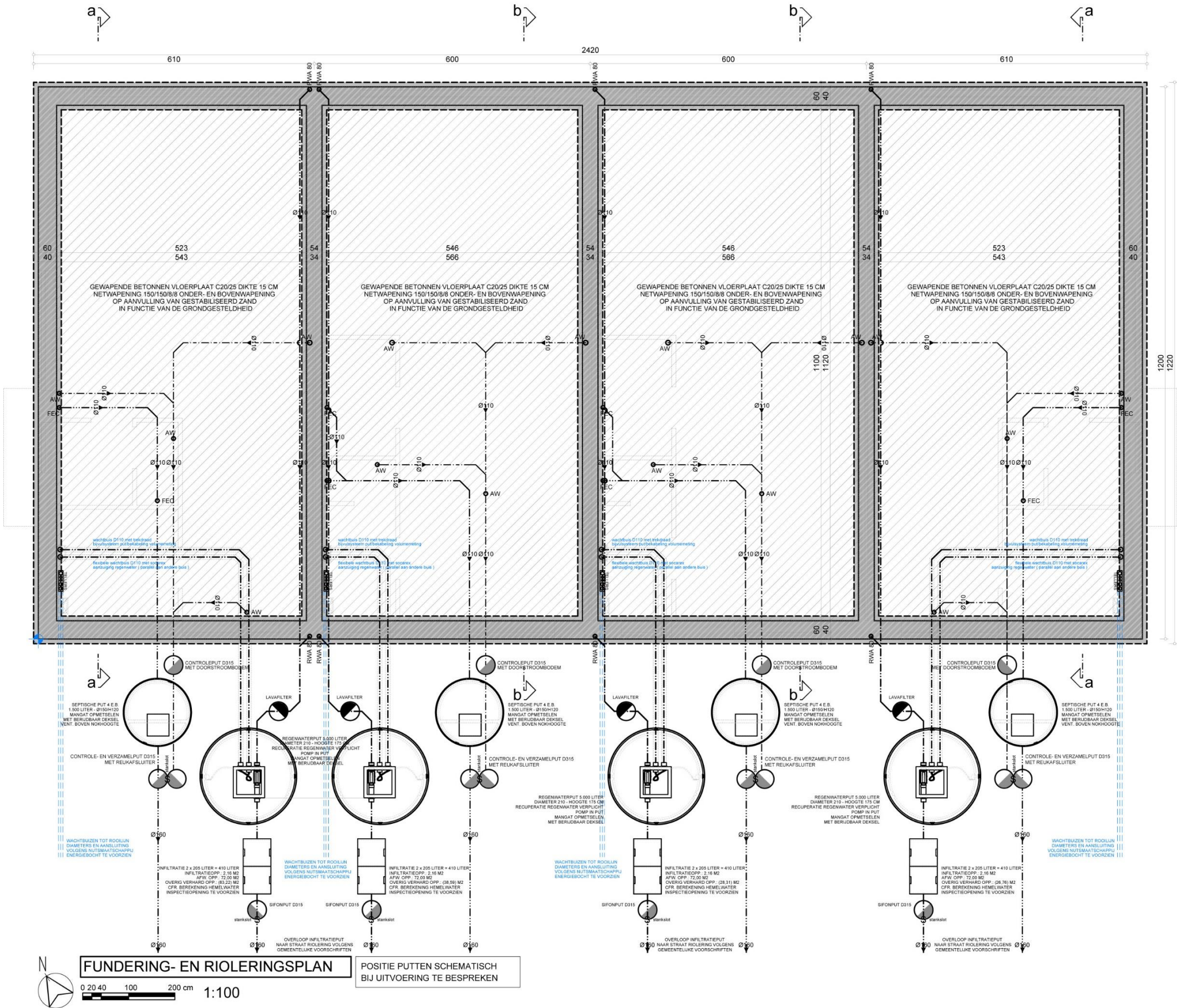
Figuur 6: Funderingsplan woningen Neerkouter
