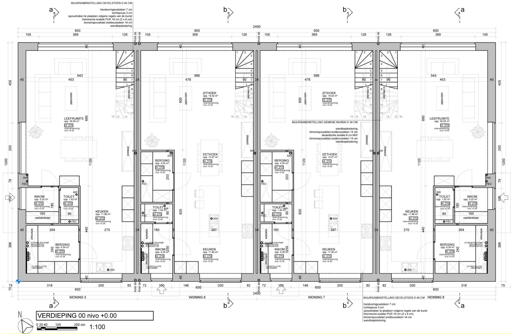
Figuur 5: Grondplan woningen Neerkouter
