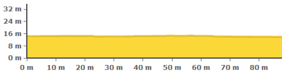
Figuur 14: Hoogteverloop van zuidwest naar noordoost over het onderzoeksgebied ( www.geopunt.be/kaart )
