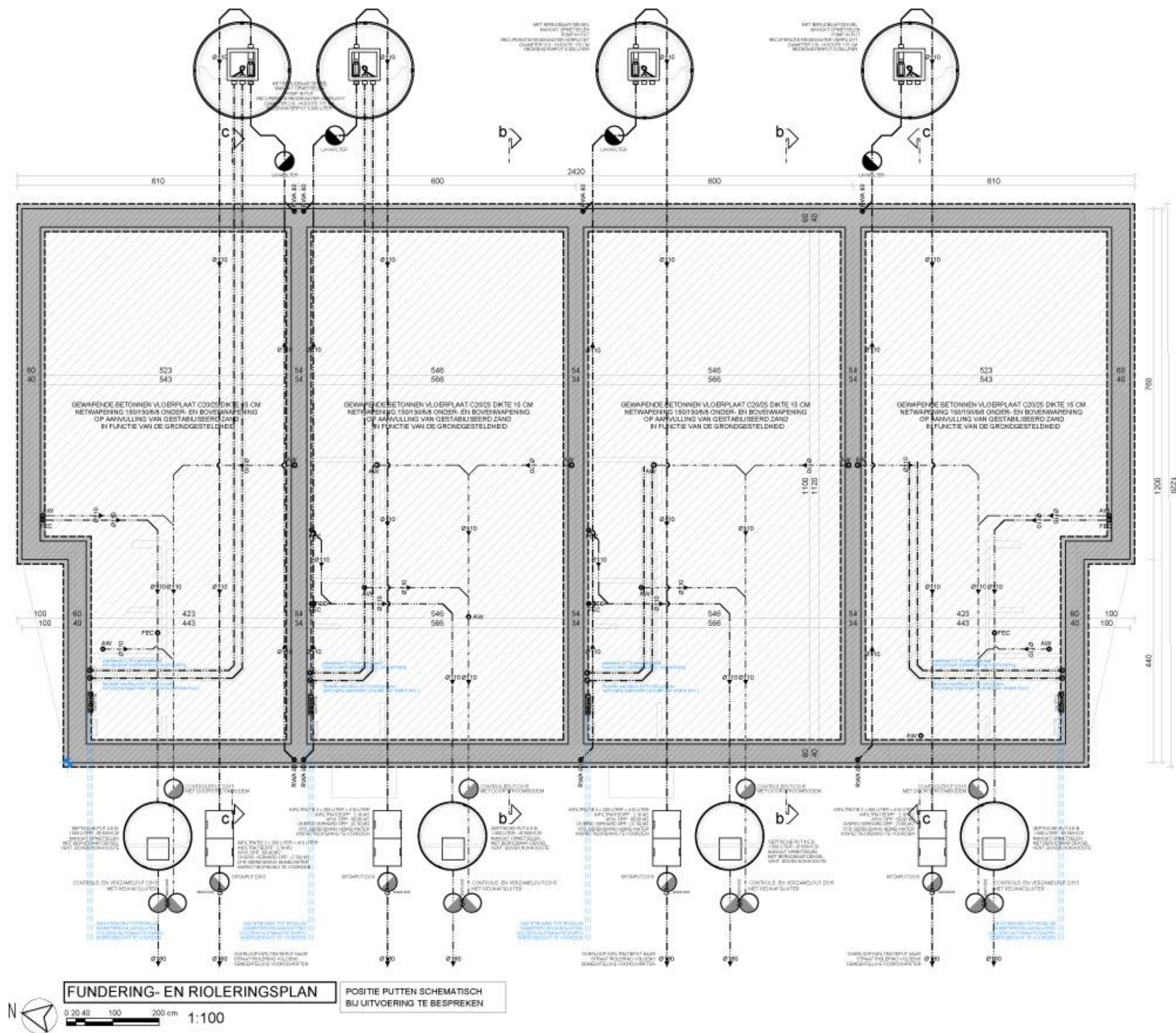
Figuur 9: Funderingsplan woningen Schrijberg
