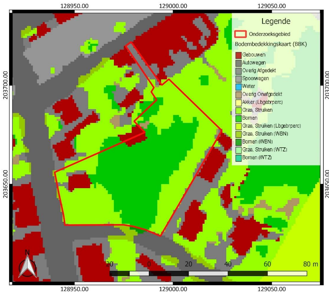
Figuur 19: Bodemgebruikskartaal met aanduiding van het onderzoeksgebied ( www.geopunt.be )
