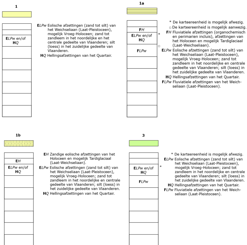
Figuur 17: Legende bij de quartairgeologische kaart ( www.geopunt.be )
