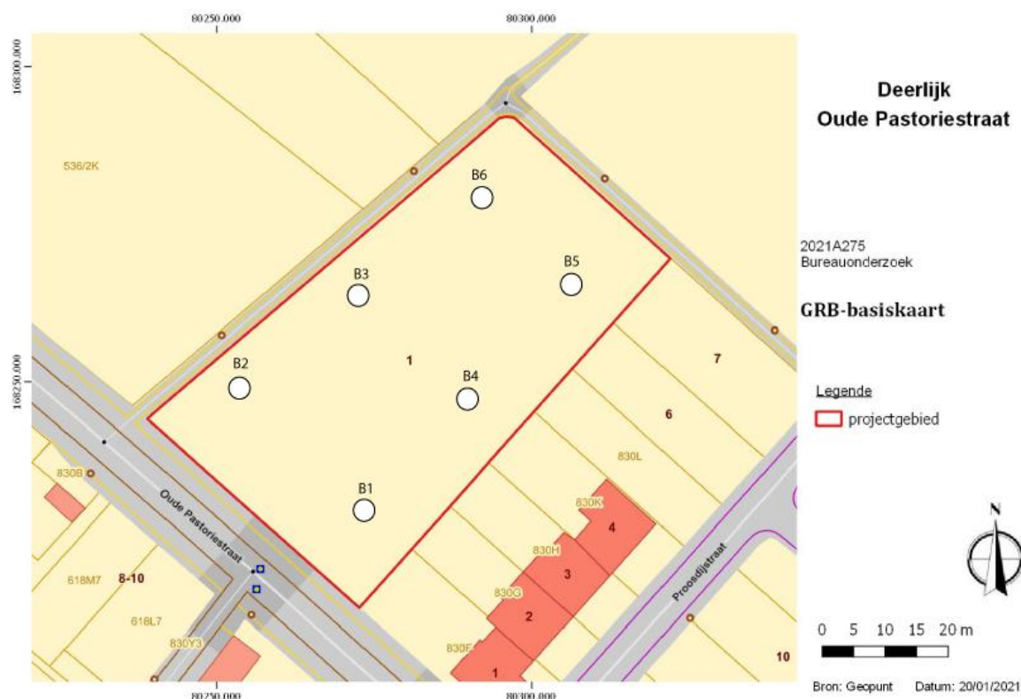
Figuur 33 Locatie van de controleboringen op de GRB-basiskaart. (bron: geopunt)
