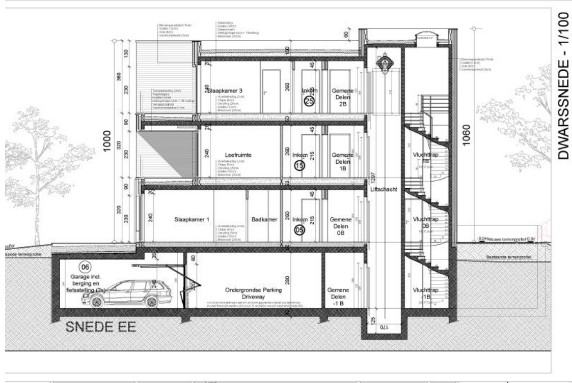
Figuur 6 Doorsnede. (bron: opdrachtgever)
