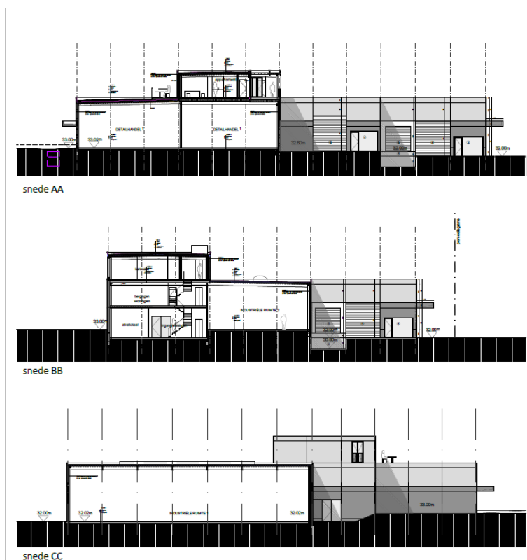
Figuur 4: Snede (initiatiefnemer, 2021)
