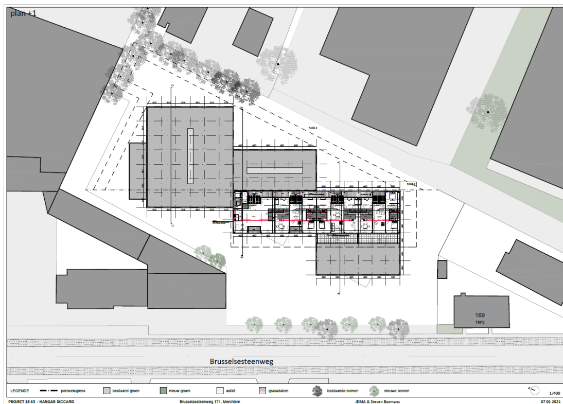
Figuur 3: Eerste verdieping (initiatiefnemer, 2021)
