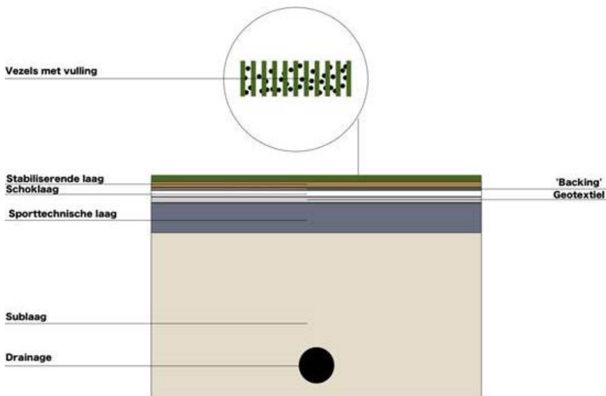
Figuur 6: Profiel van het aan te leggen kunstgrasveld 7
