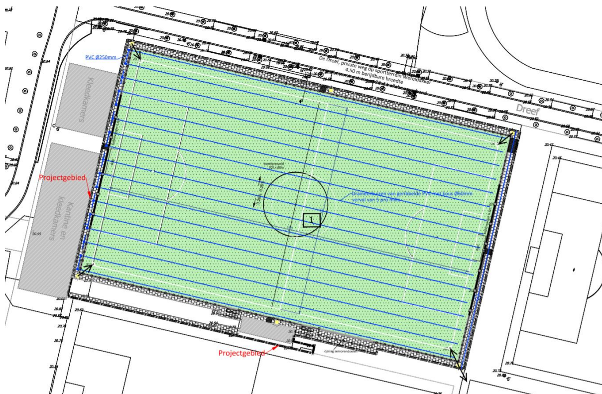
Figuur 5: Inplantingsplan 6
