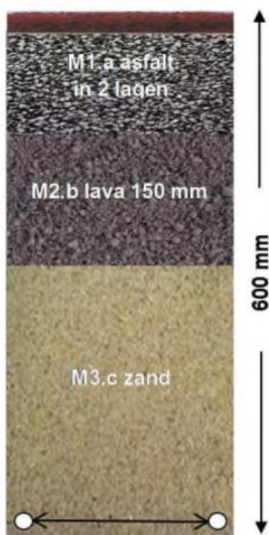
Figuur 7: Opbouw atletiekpiste
