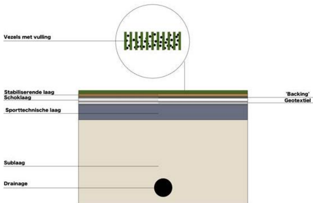
Figuur 6: Profiel van het aan te leggen kunstgrasveld 7
