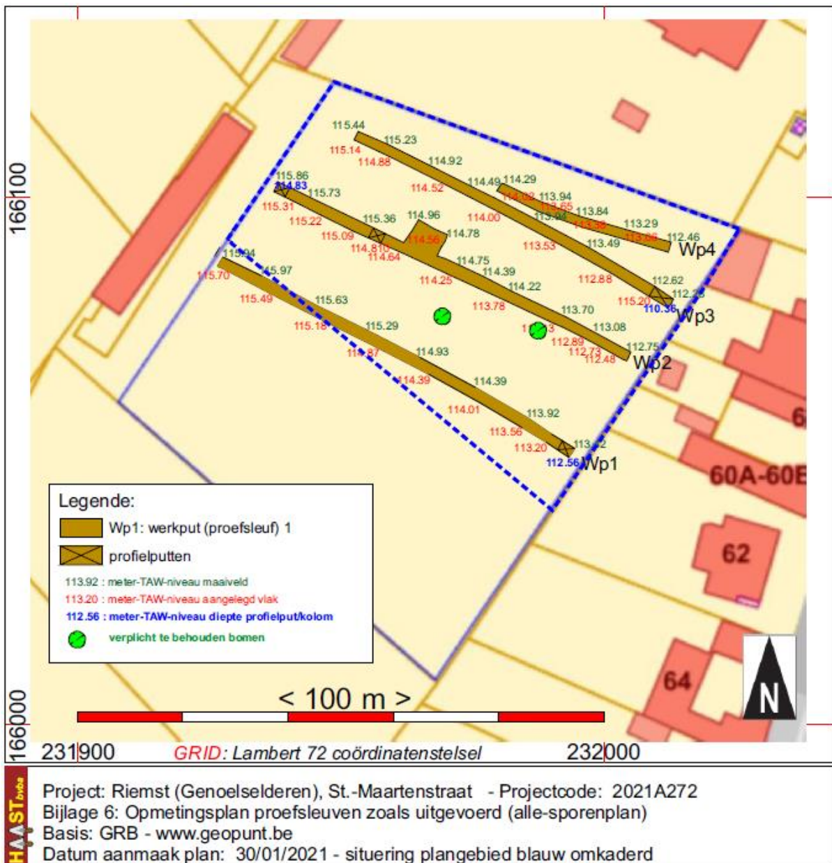
Fig. 1: opmetingsplan van het uitgevoerd proefsleuvenonderzoek
