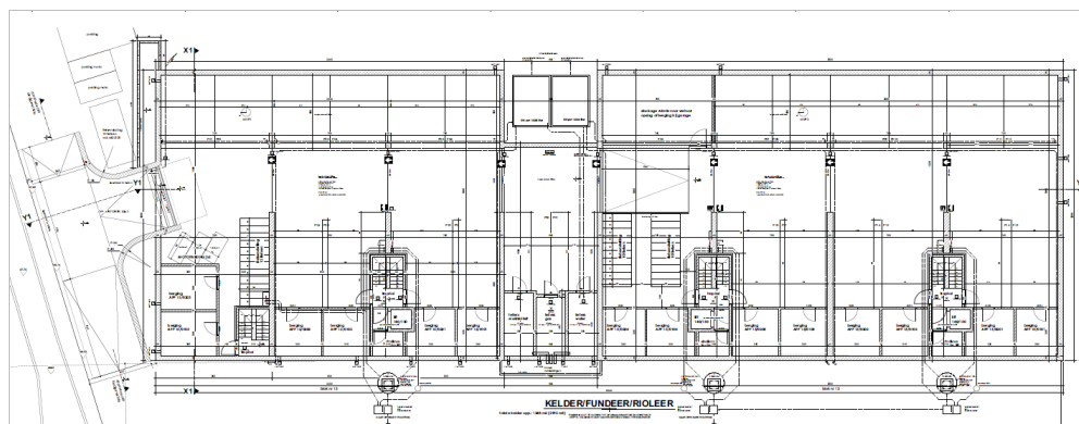
Figuur 3: Kelder-fundering-riolering (Herman De Becker, 2021)
