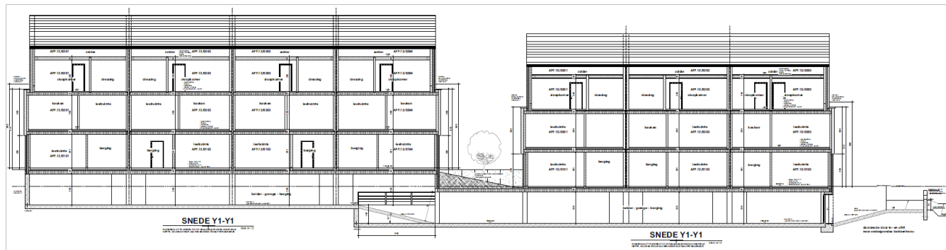
Figuur 4: Snede Y1-Y1 (Herman De Becker, 2021)
