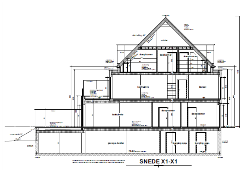
Figuur 5: Snede X1-X1 (Herman De Becker, 2021)
