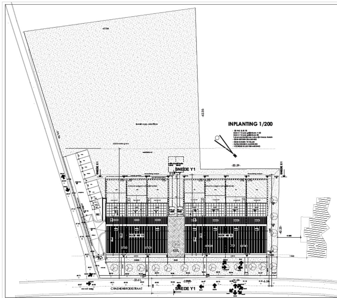
Figuur 2: Inplanting (Herman De Becker, 2021)
