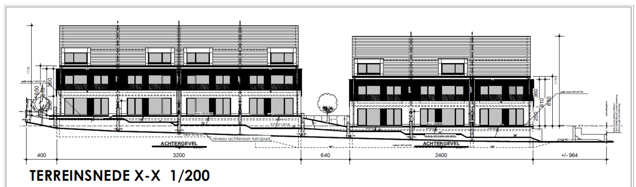
Figuur 6: Terreinsnede X-X (Herman De Becker, 2021)
