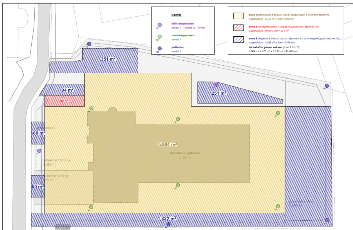
Figuur 2 Uitsnede uit het grondverzetplan: geel = afgraven tot 1m diep, blauw = afgraven tot 2m diep, rood = afgraven tot 3m diep (bron: initiatiefnemer).
