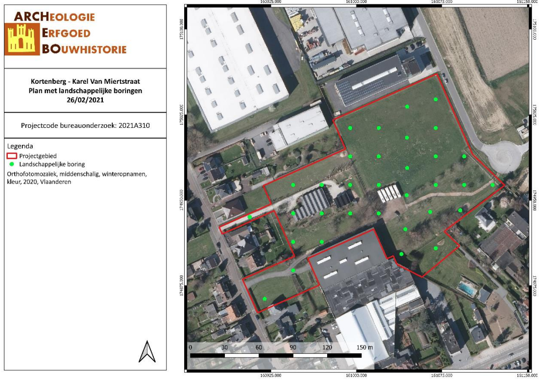
Figuur 6: Locatie boorpunten op het onderzoeksterrein (ARCHEBO bvba, 2021)
