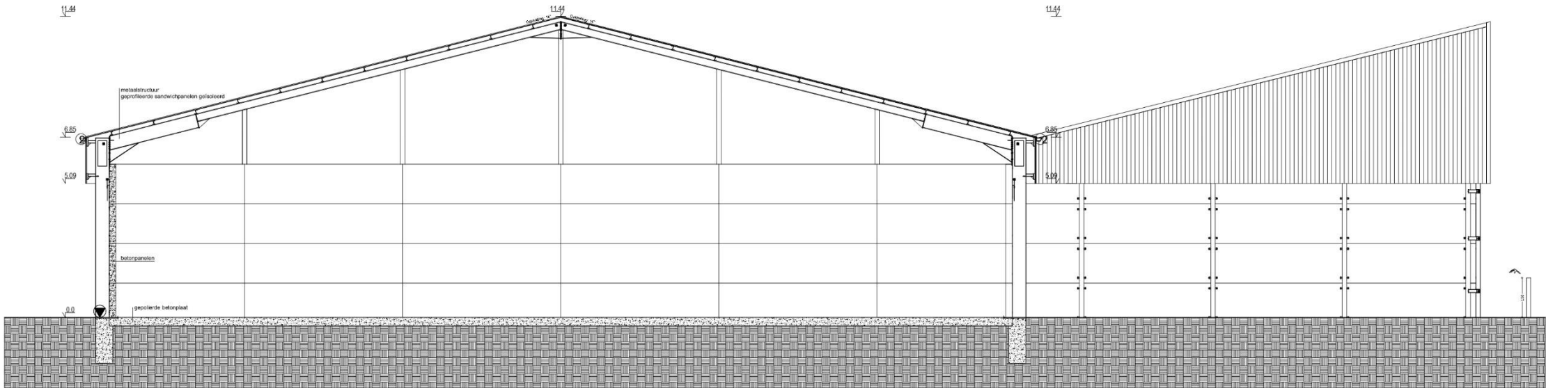
Doorsnede AA
