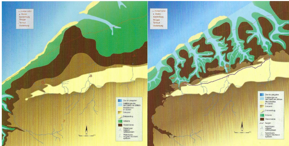
Figuur 5. Evolutie van de kustvlakte vanaf het Neolithicum tot de IJzertijd 7
