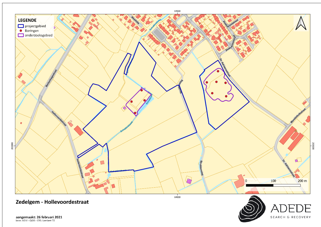
Figuur 3. Boorplan
