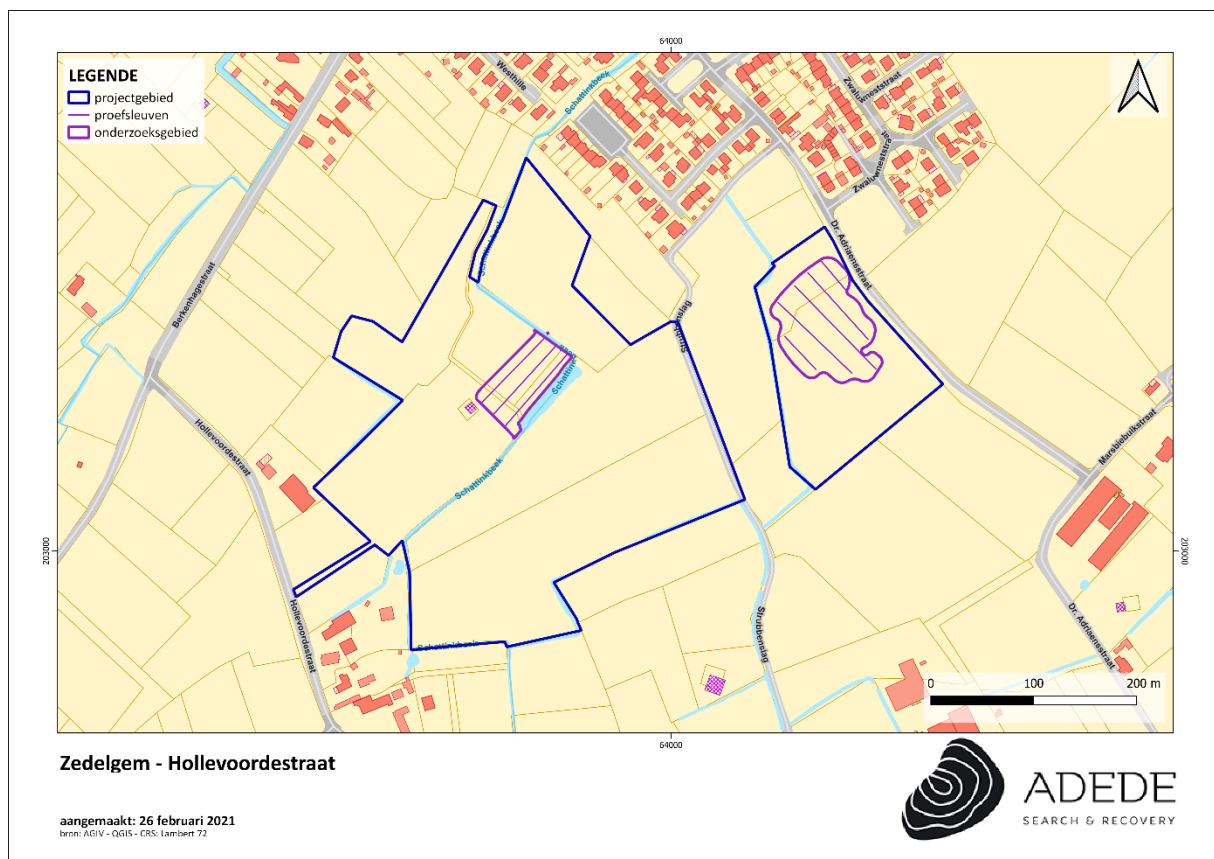
Figuur 4. Proefsleuvenplan
