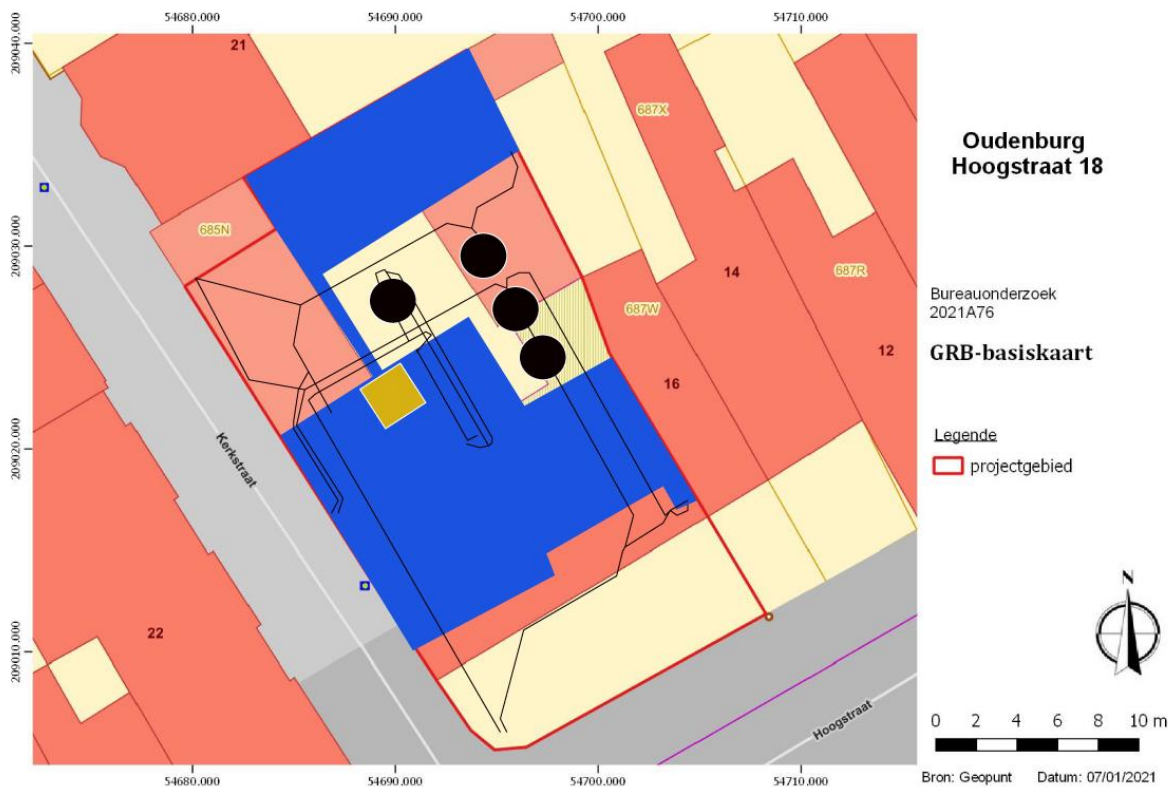
Figuur 1 Vereenvoudigde weergave van de geplande werken op de GRB-basiskaart. Legende: blauw: nieuwbouw, geel: liftkoker, zwarte ronde: putten, zwart lijn: riolering. (Bron: geopunt)
