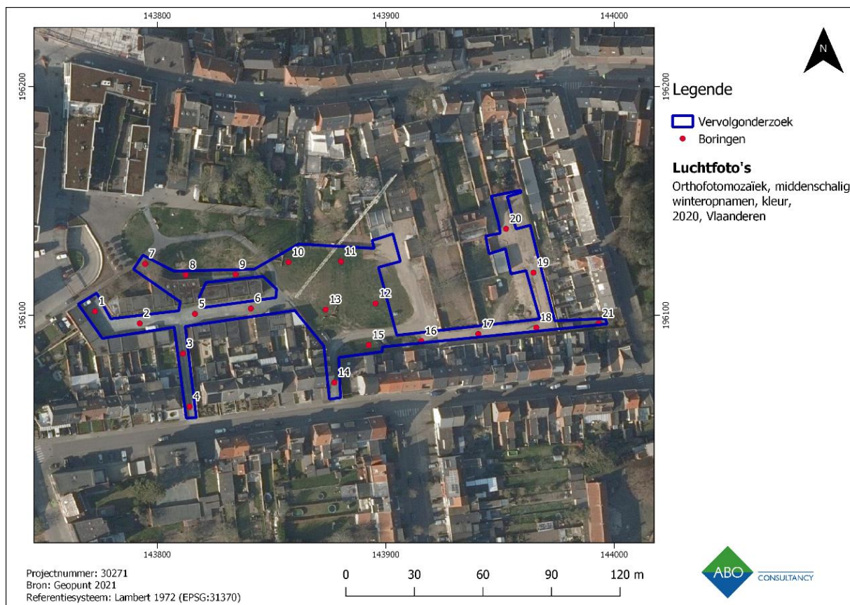
Figuur 2: Luchtfoto (2020) met aanduiding van het boorplan.
