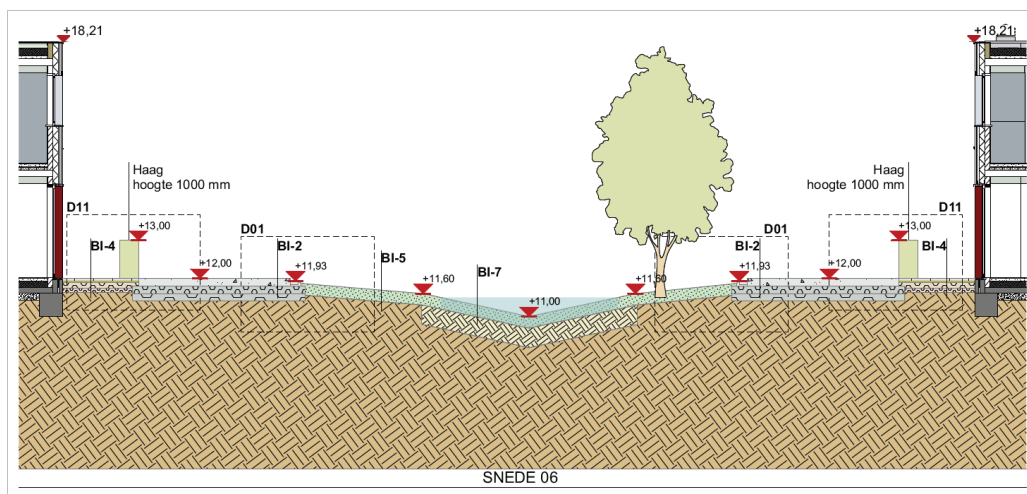
Figuur 9: Snede (opdrachtgever, 2021)
