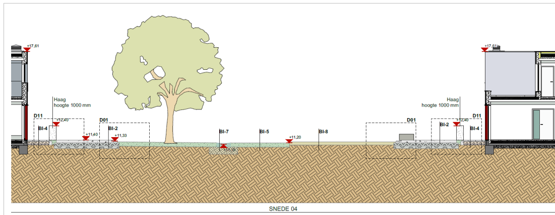
Figuur 7: Snede (opdrachtgever, 2021)
