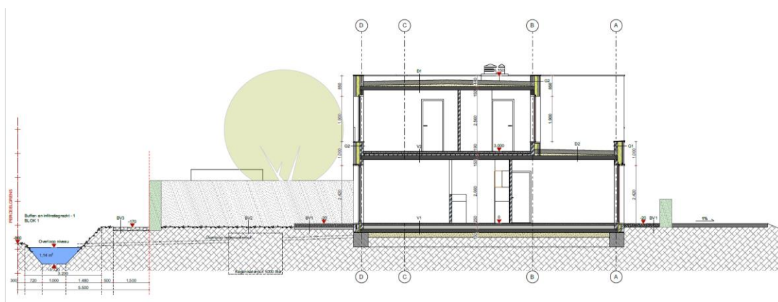
Figuur 10: Snede gebouw (opdrachtgever, 2021)
