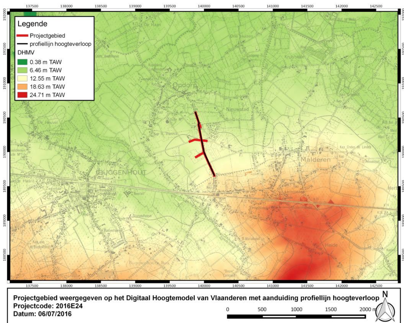
Figuur 10: Projectgebied weergegeven op het Digitaal Hoogtemodel van Vlaanderen met aanduiding van de profiellijn van het hoogteverloop (bron: Geopunt).
