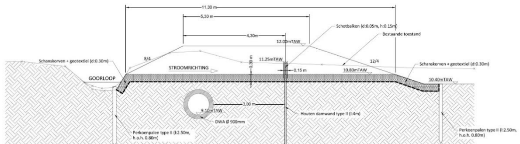
Figuur 15: doorsnede inlaatconstructie uit hout op het oostelijke deel van het projectgebied
