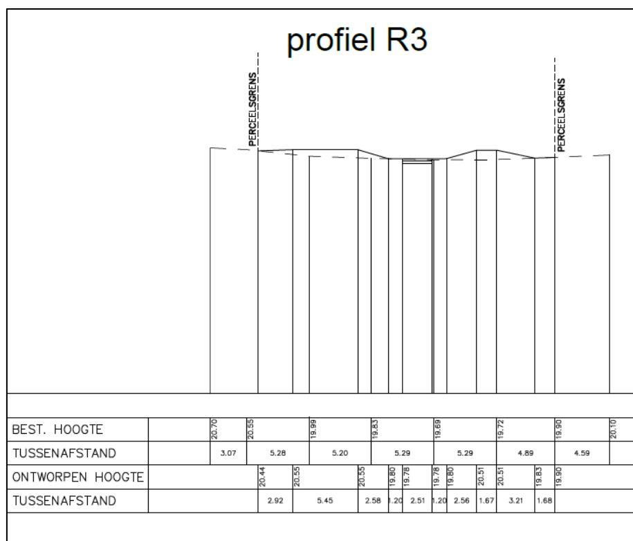
Figuur 10: Ontwerp reliëfaanpassingen doorsnede (initiatiefnemer 2021).
