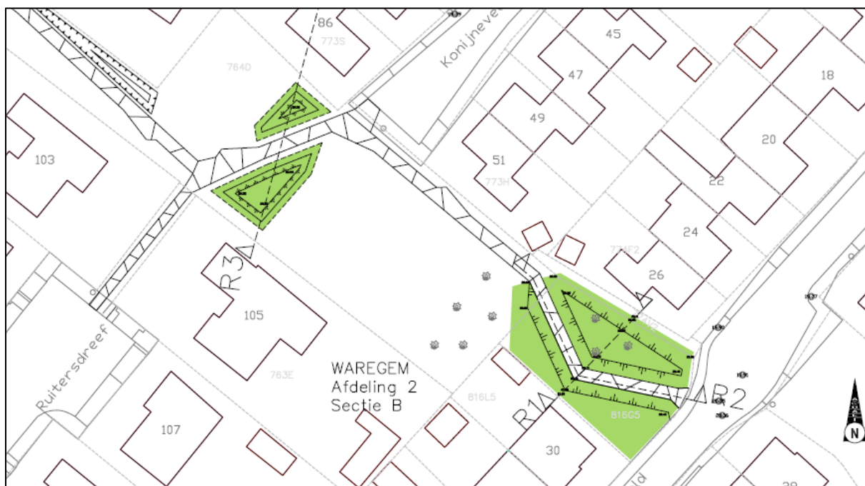
Figuur 9: Ontwerp reliëfaanpassingen (initiatiefnemer 2021).
