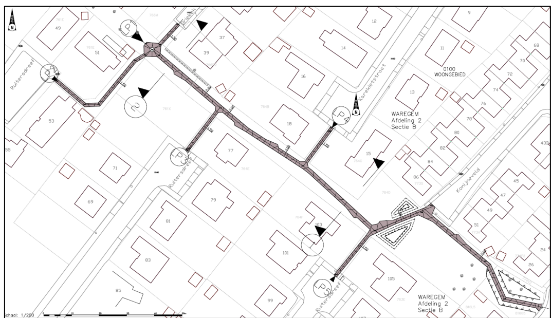
Figuur 11: Ontwerp nieuwe verharding (initiatiefnemer 2021).
