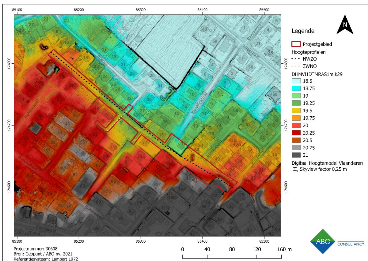
Figuur 16: Digitaal Hoogtemodel (DHM VII) (1m) en Skyview (0,25m) met aanduiding van het projectgebied en de waterlopen: detail.
