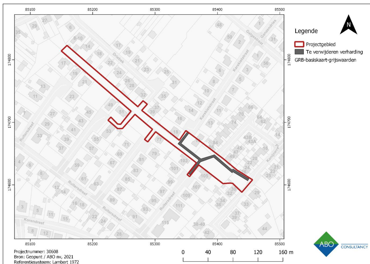
Figuur 12: Toekomstplan, locatie uit te breken verharding.
