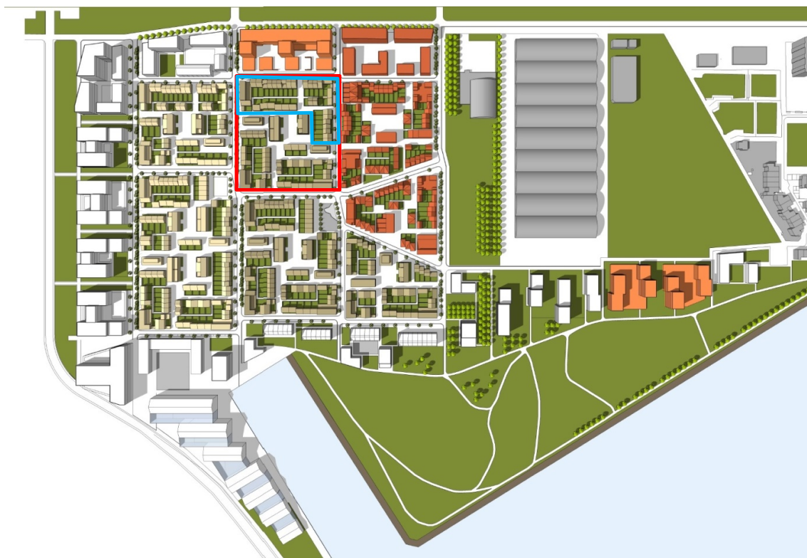
figuur 4 Overzicht van het totaalplangebied Regatta met in het rood en oranje de reeds gerealiseerde bouwblokken. Binnen het rode kader wordt de deelzone Wijk 4 aangegeven, in blauw de zone waarvoor nu een stedenbouwkundige vergunning voor wordt aangevraagd. (Naar: actualisatie inrichtingsplan januari 2015, awg architecten, p. 16-17).
