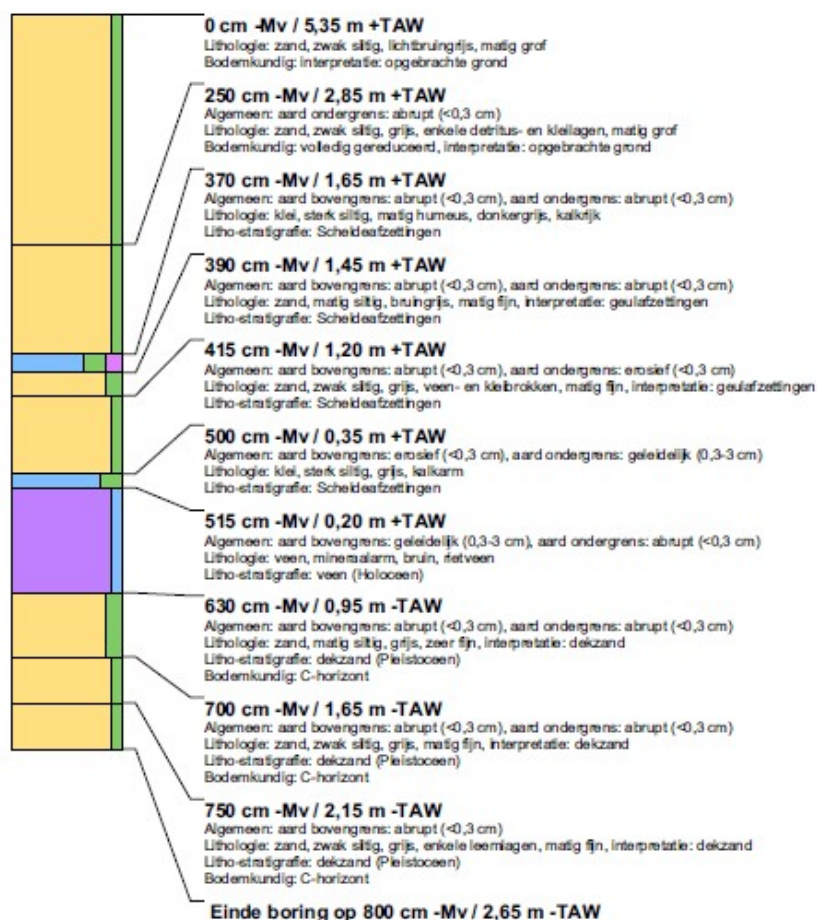
figuur 12 Bodemprofiel van boring 17 (noordwesthoek van deelzone Wijk 4 – deel 1) (uit: Smits & Timmerman, 2010, 54).
