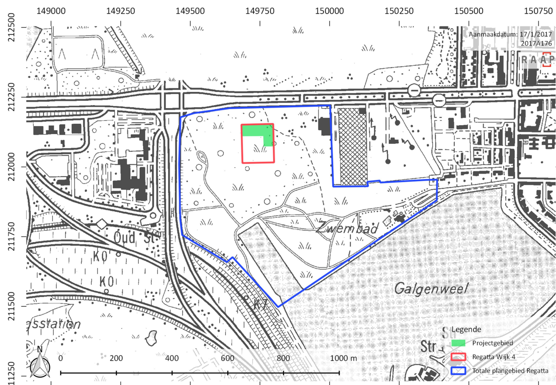
figuur 1 Topografische kaart met projectie van het plangebied (bron: NGI) (schaal 1:12 500).
