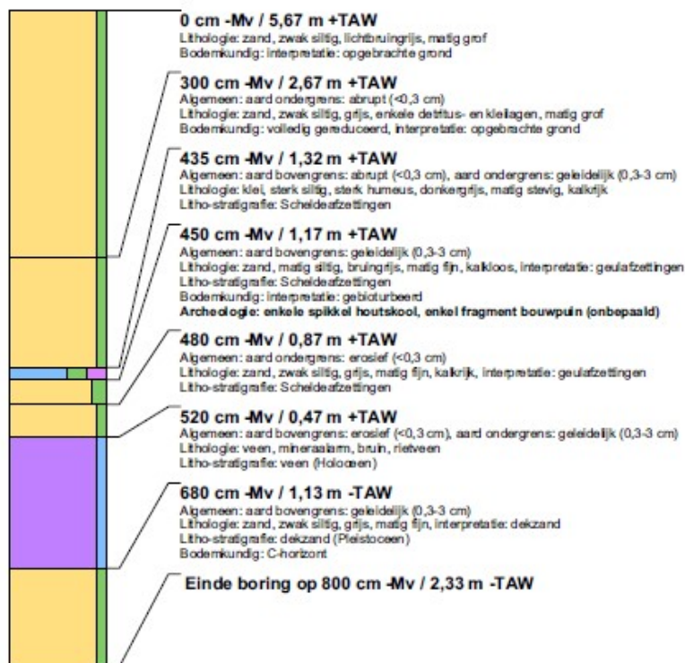
figuur 13 Bodemprofiel van boring 31 (in het oosten van deelzone Wijk 4 – deel 1) (uit: Smits & Timmerman, 2010, 76).
