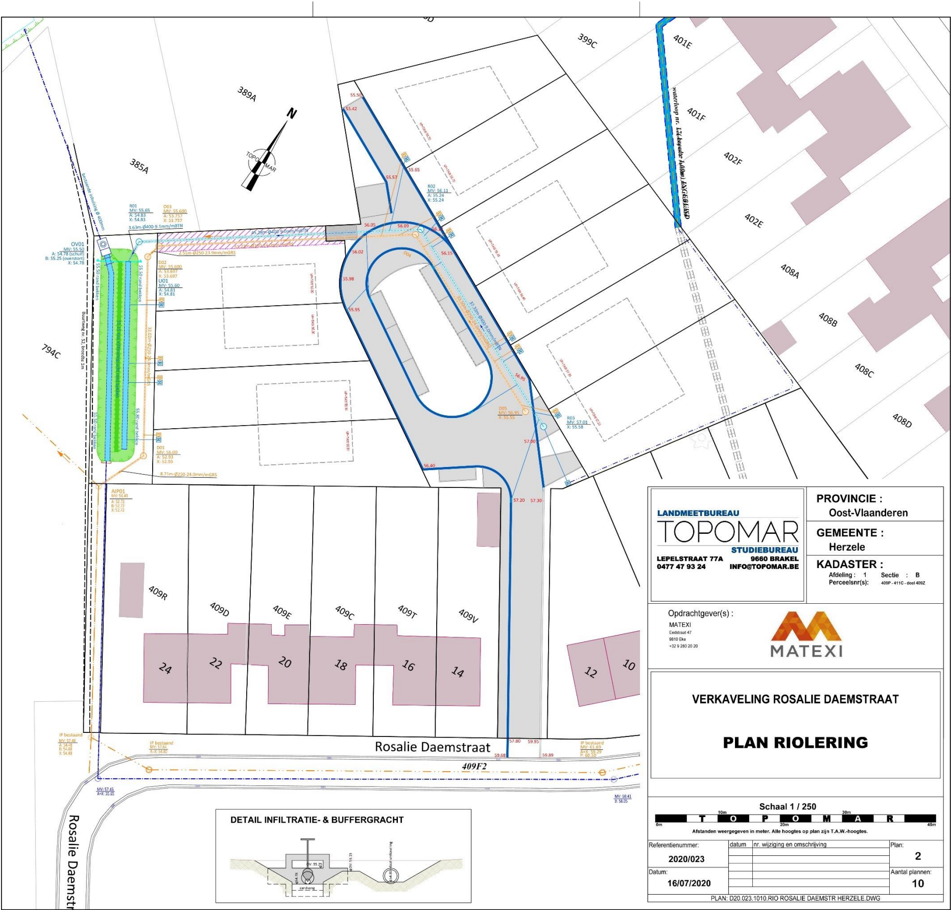
Figuur 3: Ontwerpplan (Topomar)
