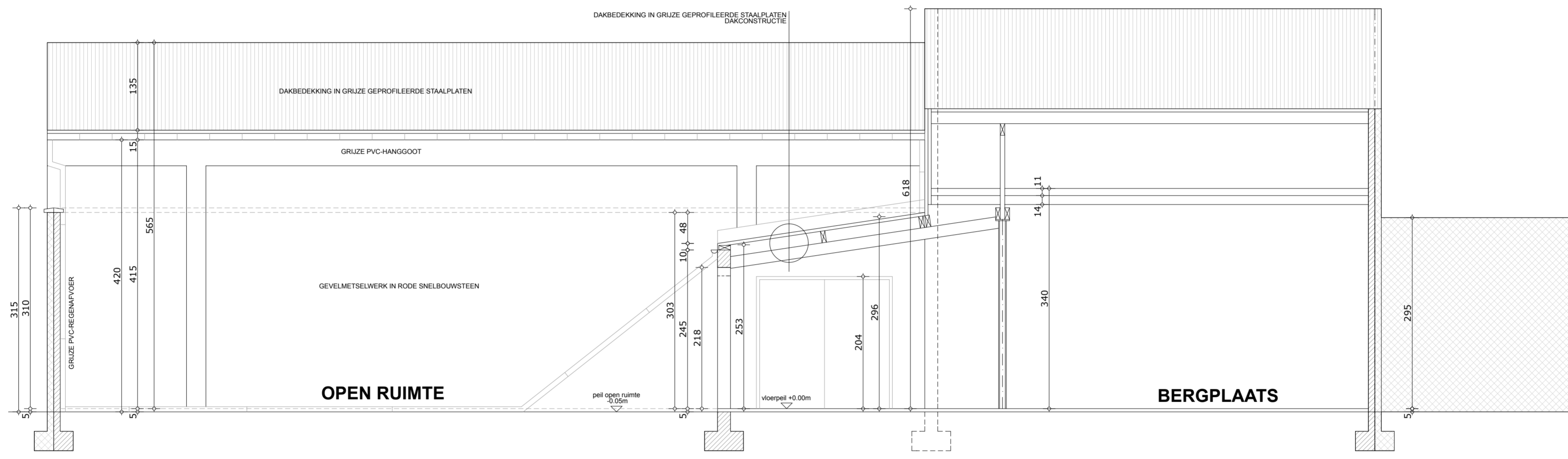
DOORSNEDE AB - BESTAANDE TOESTAND SCHAAL 1-50
