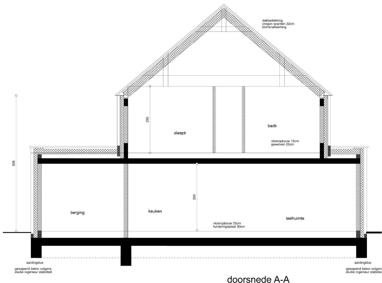
Figuur 3.4 : Dwarsdoorsnede van het geplande bouwproject.
