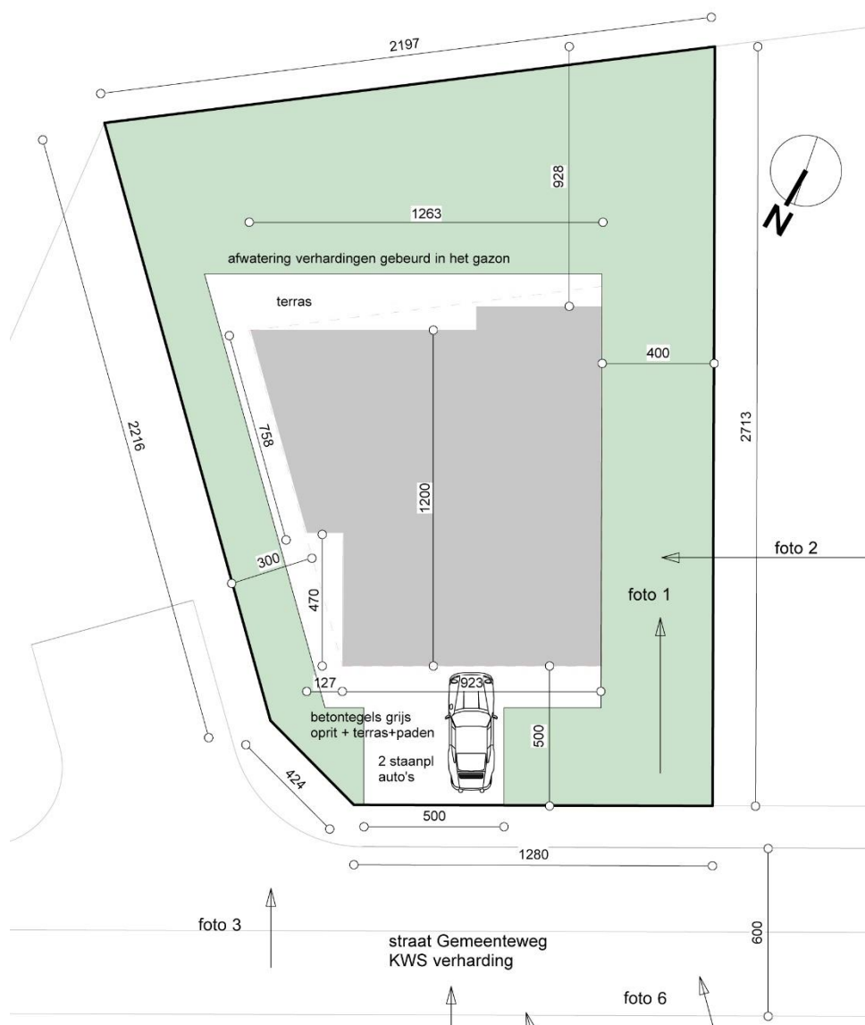
Figuur 3.2 : Grondplan van het geplande bouwproject.
