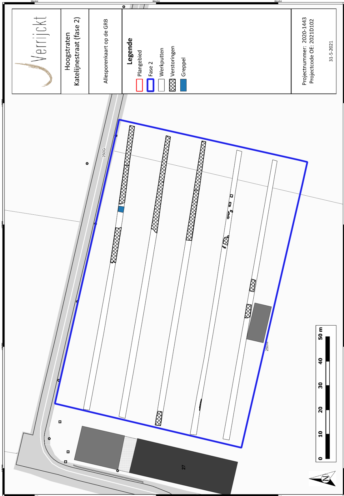
Figuur 1: Syntheseplan.
