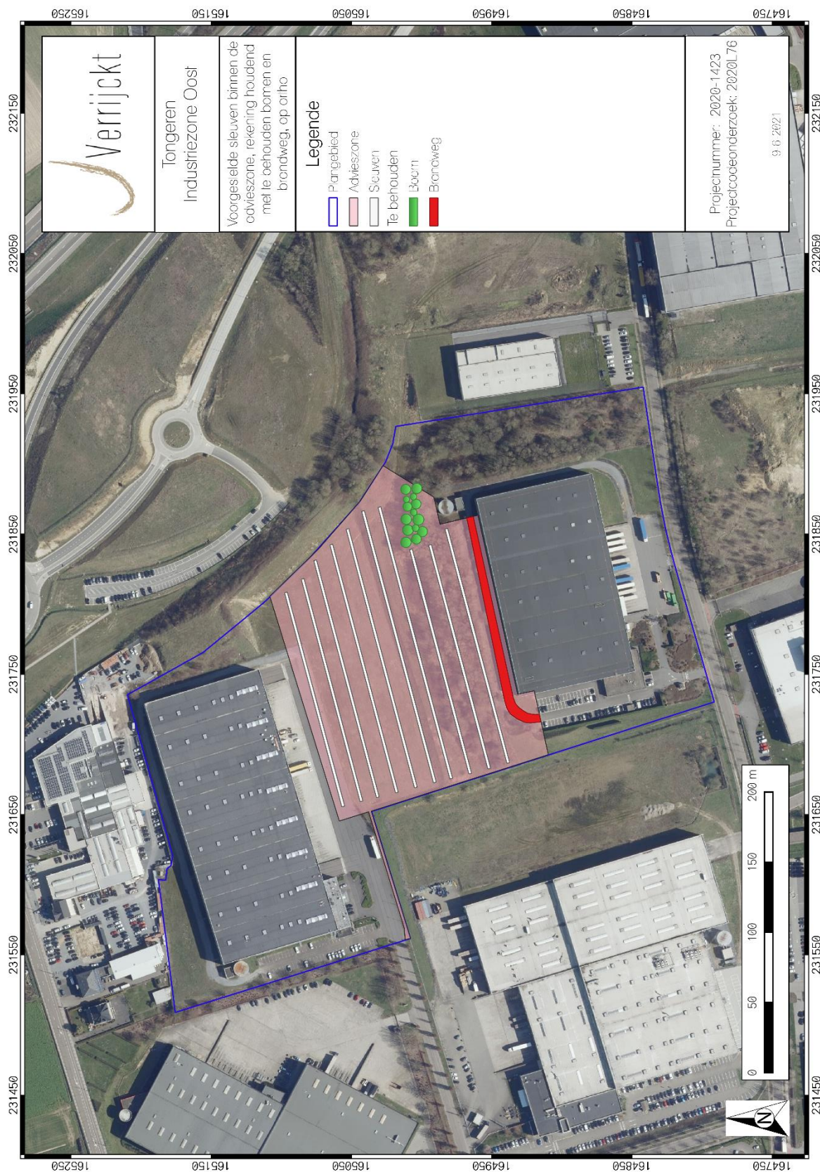
Figuur 3: Sleuvenplan op orthofoto, rekening houdend met te behouden bomen (groen) en brandweg (rood)
