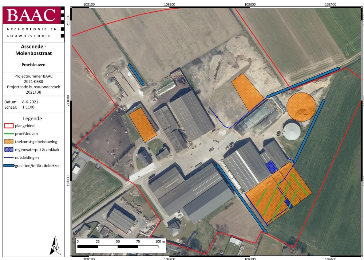
Plan 2: Inplanting proefsleuven (digitaal; 1:1; 08.06.2021)
