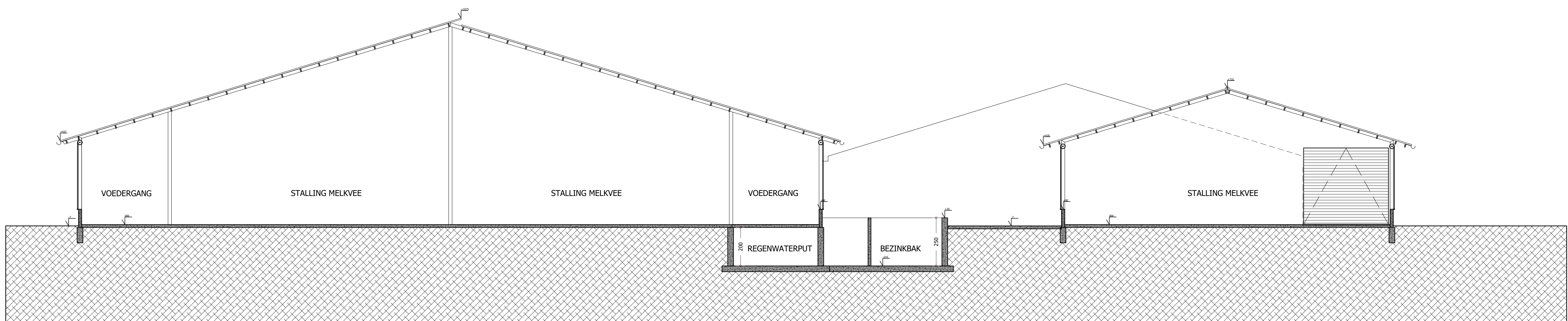
MELKVEESTAL SNEDE 1/100
