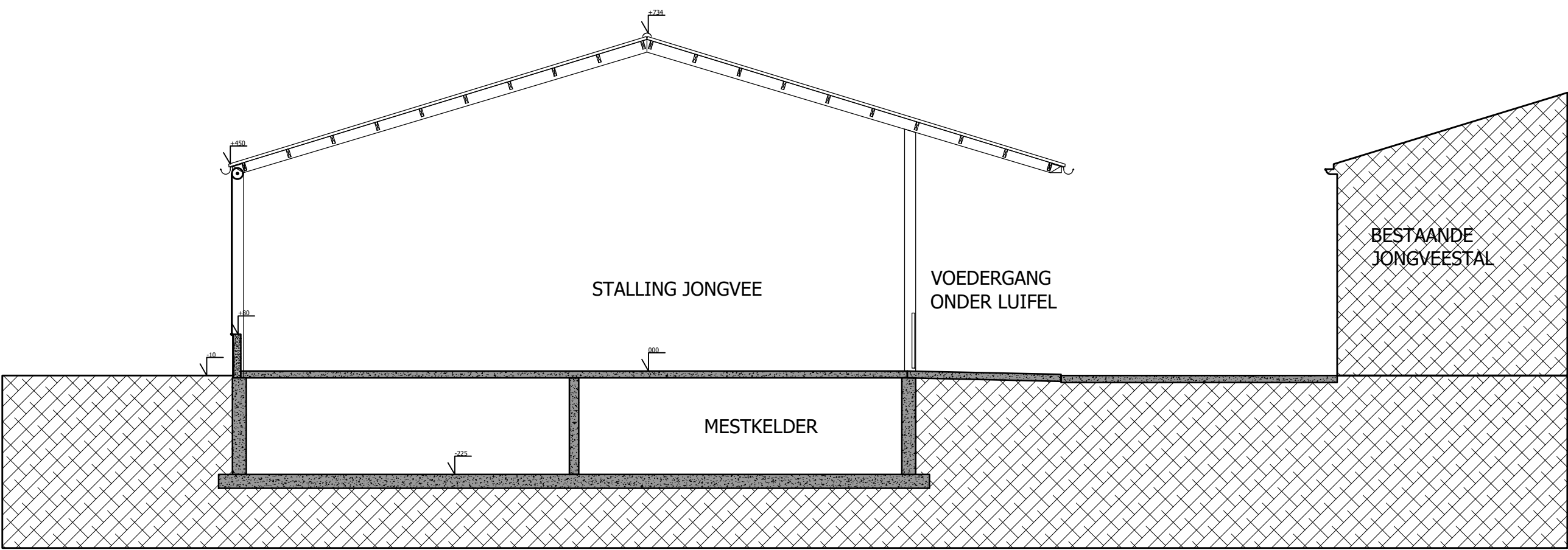
JONGVEESTAL SNEDE 1/100
