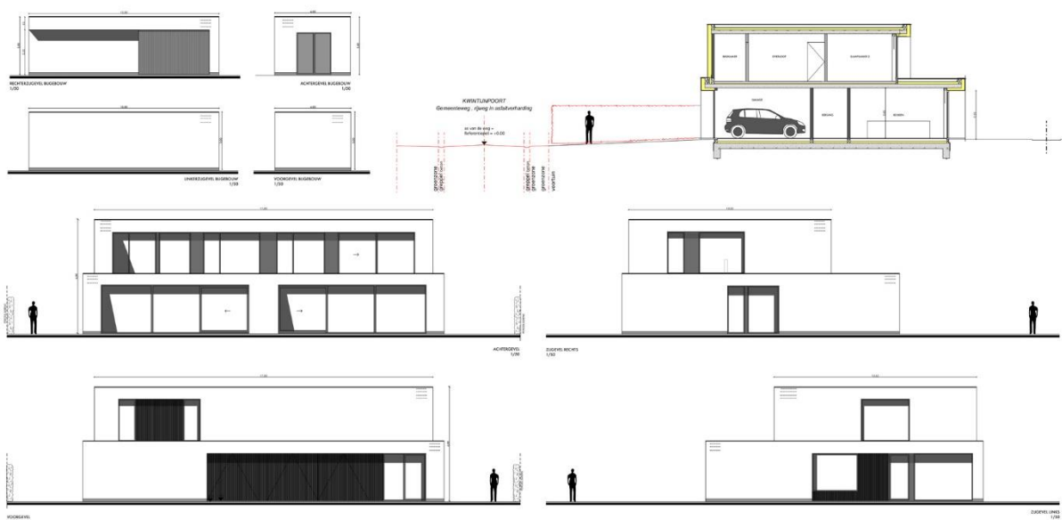
Figuur 2.5a: Opgaande plannen van de geplande woningen.
