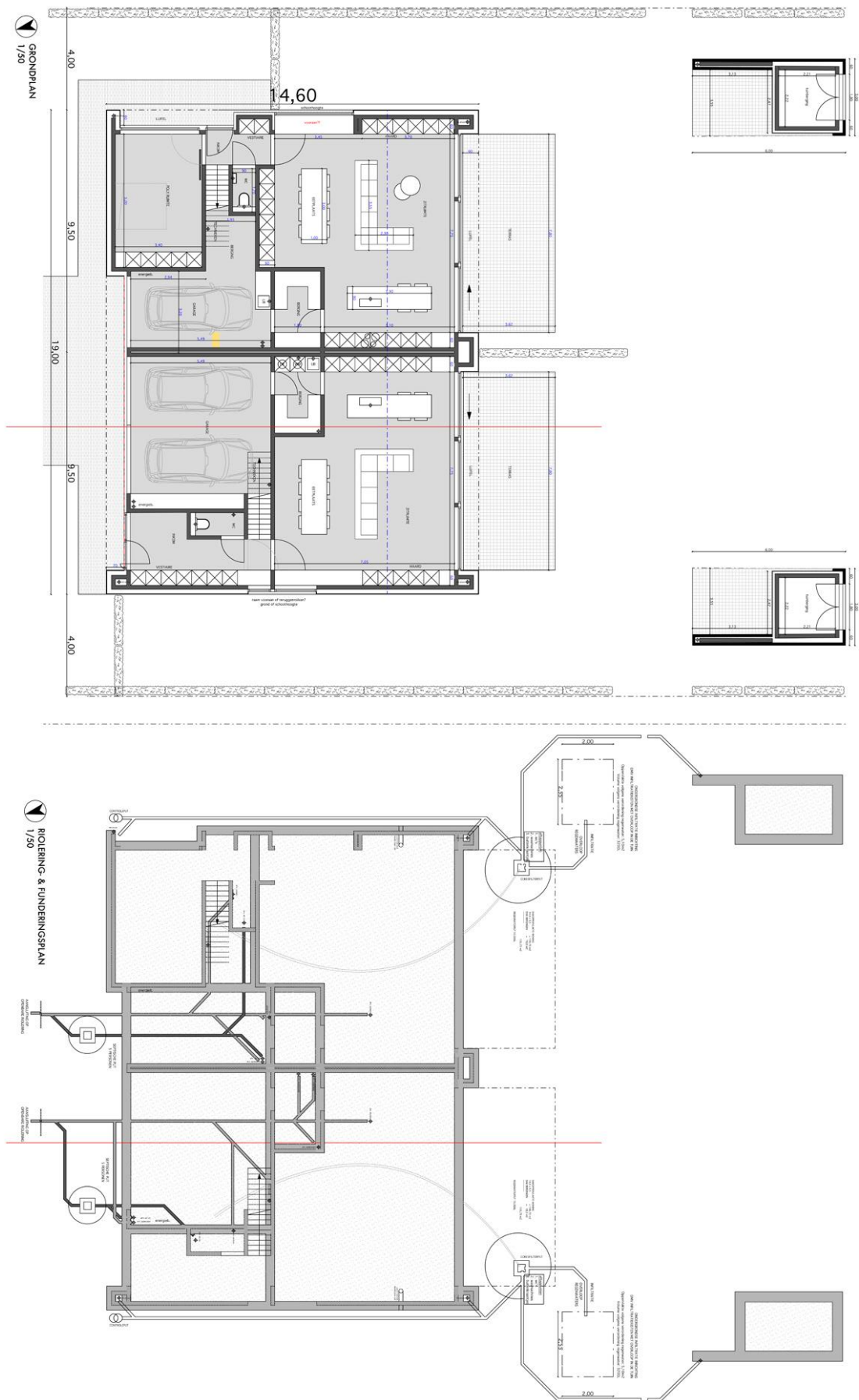
Figuur 2.5b: riolerings- en funderingsplan (onder) en grondplan (boven) van de geplande bebouwingen.
